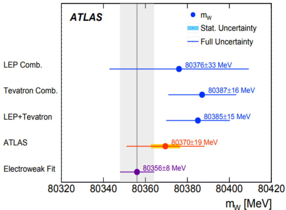
图 2：W 玻色子的质量的实验测量值比电弱拟合值的比较。
