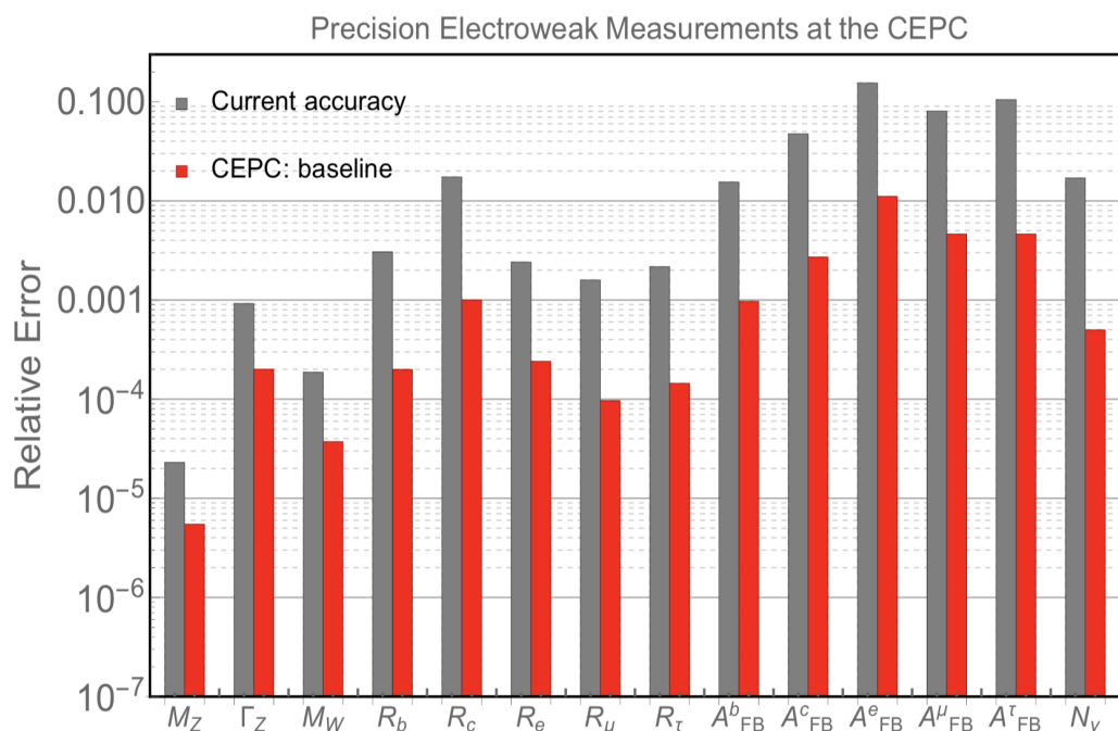
图 1：CEPC 电弱物理观测量的预计测量精度和现有测量精度对比
