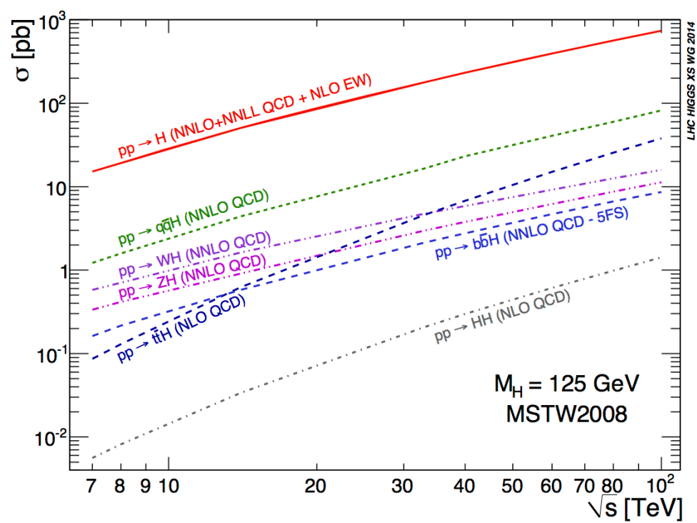
图 1.1: 强子对撞中希格斯粒子的产生截面 [?].
