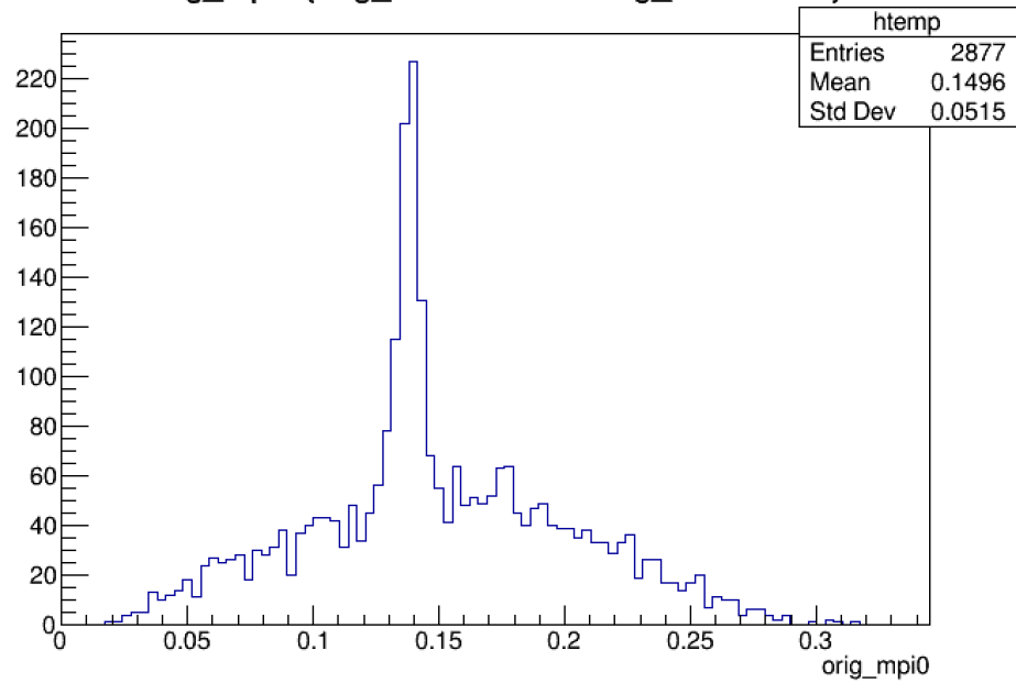
orig_mpi0 {orig_meta<0.56&&orig_meta>0.53}
