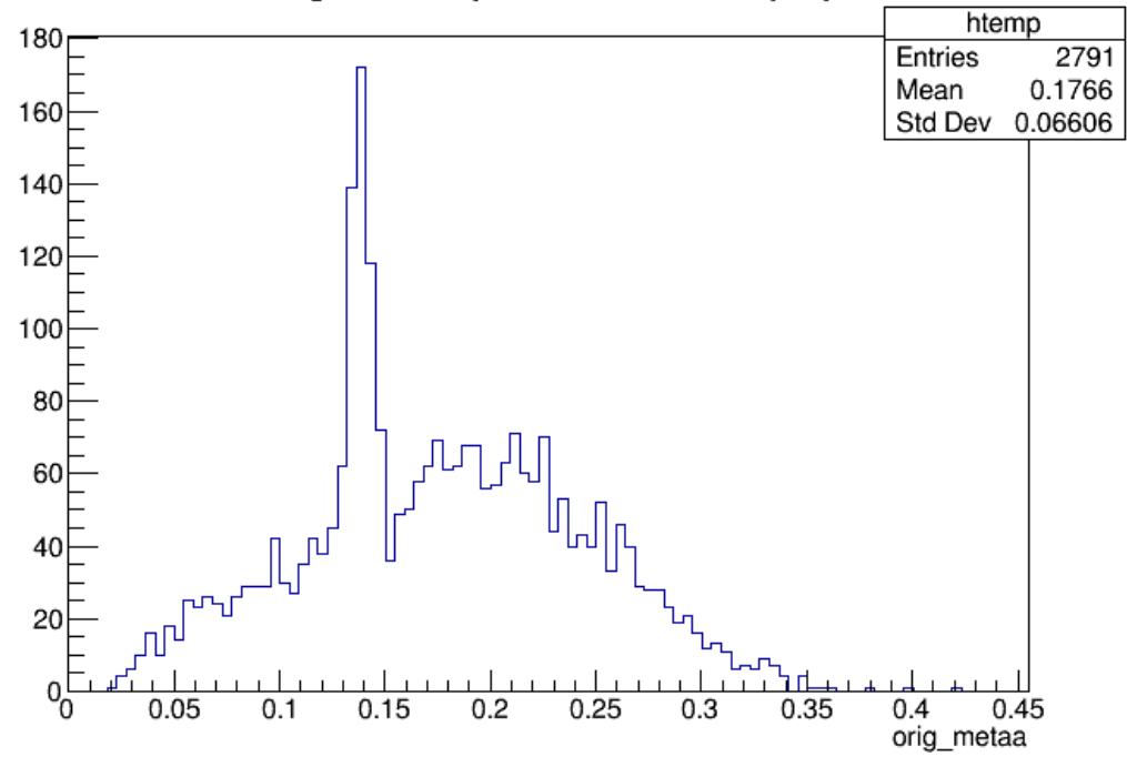
orig_metaa {delta_eta&lt;delta_pi0}
