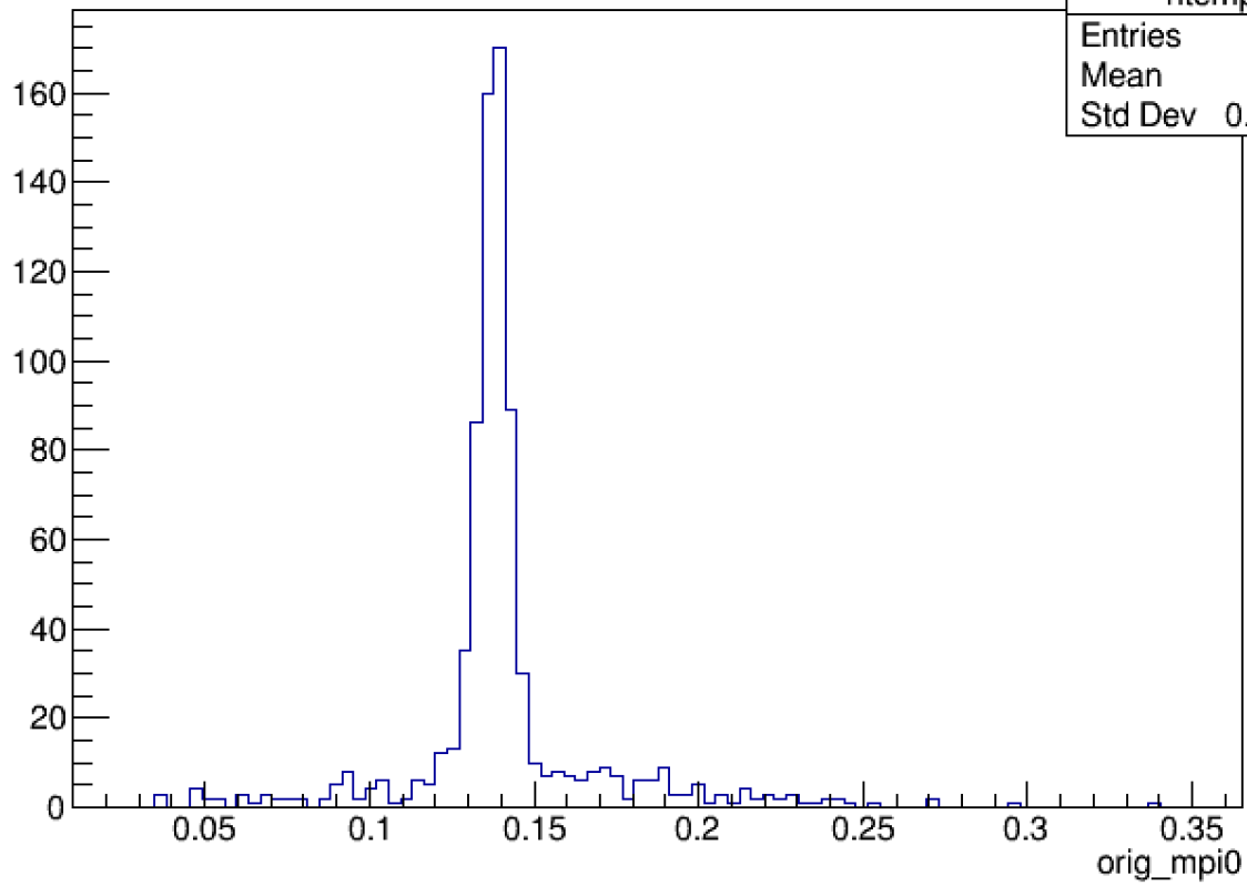
orig_mpi0
