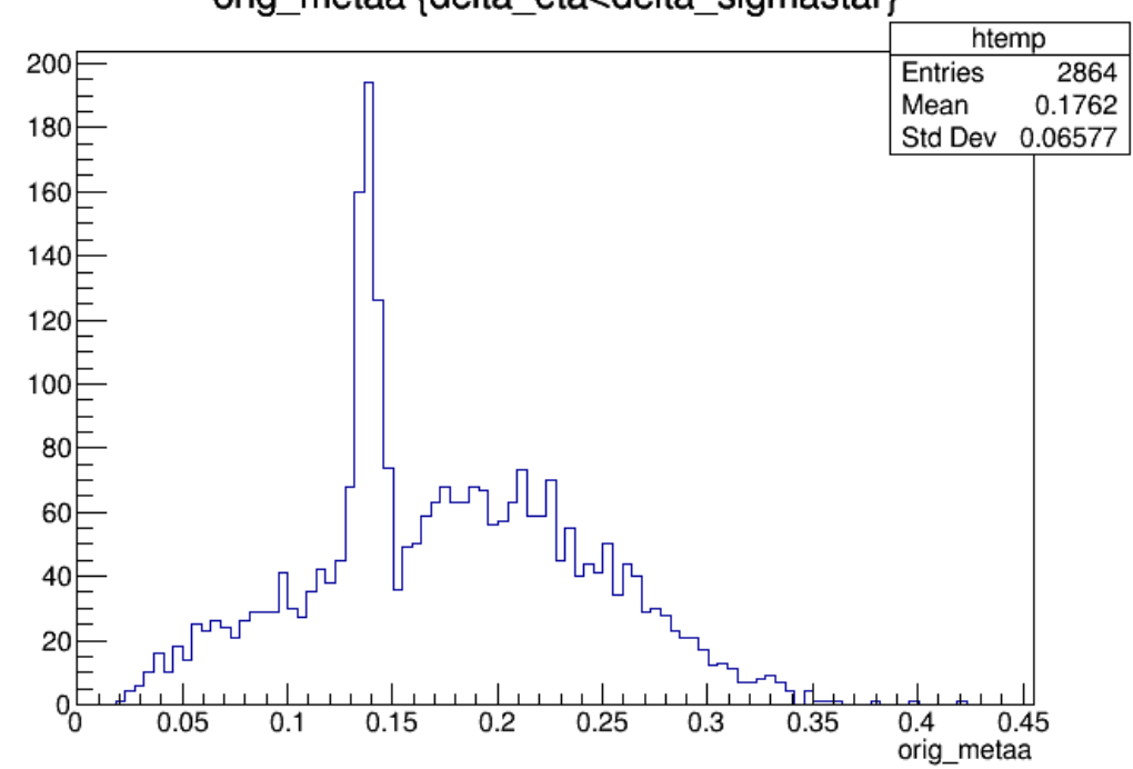
orig_metaa {delta_eta&lt;delta_sigmastar}
