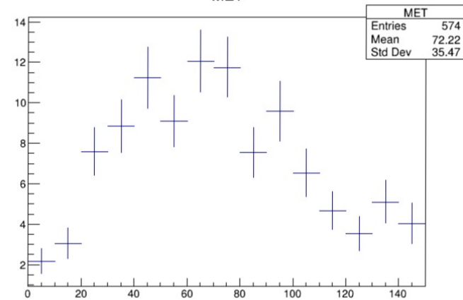
MET
