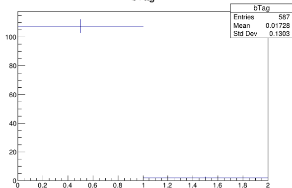
bTag
