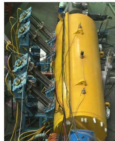
SSC-Linac 4- Rod RFQ
