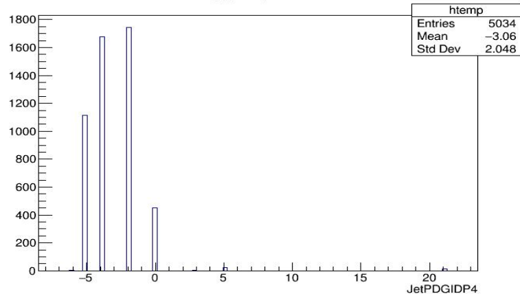
JetPDGIDP4
