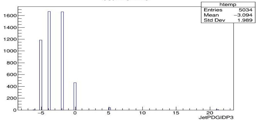
JetPDGIDP3
