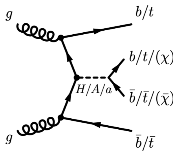
t\bar{t}t\bar{t}
