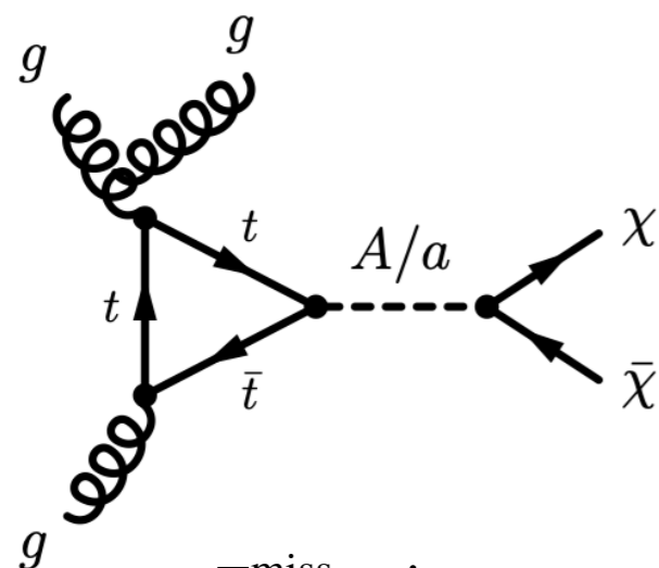
E_T^{\text{miss}} + \text{jet}
