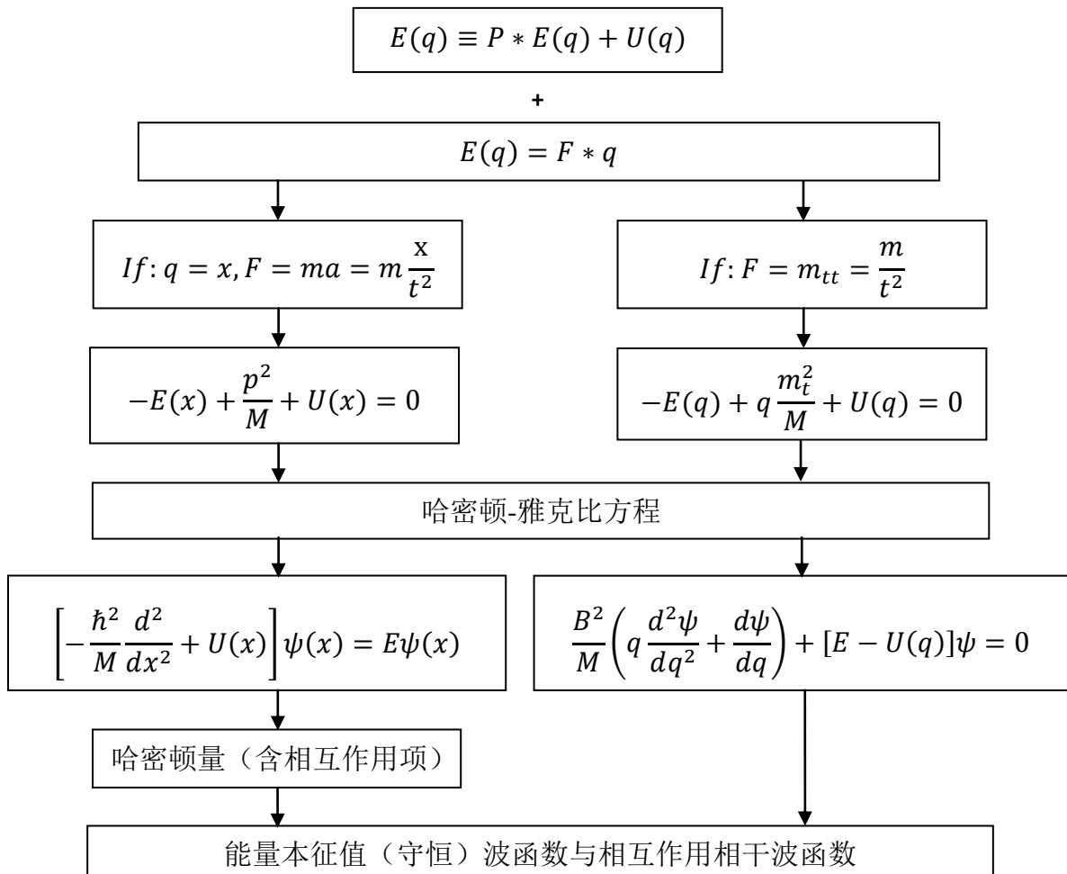
图 8 薛定谔波动方程与非定域量子波动方程的统一范式
