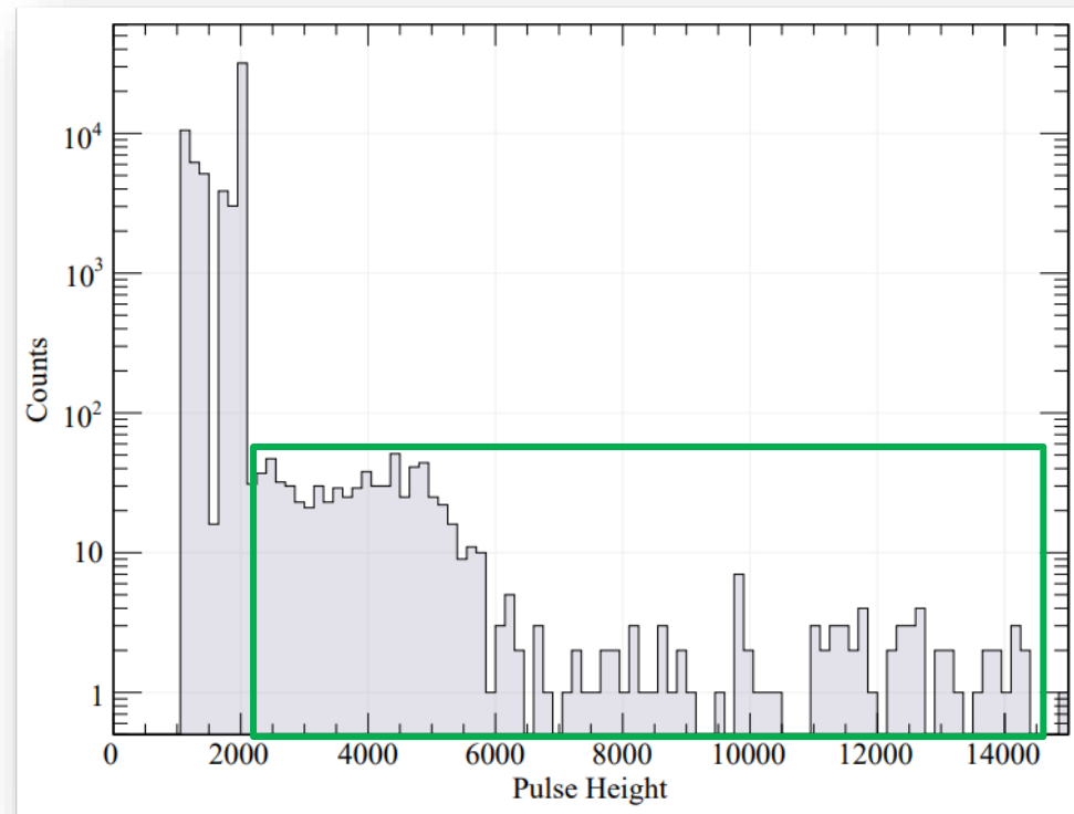
宇宙线测试
