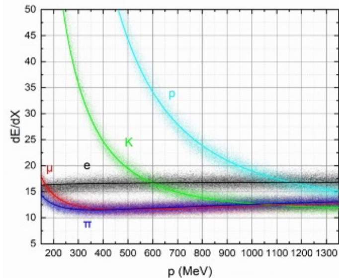
dE/dx 分辨性能.
