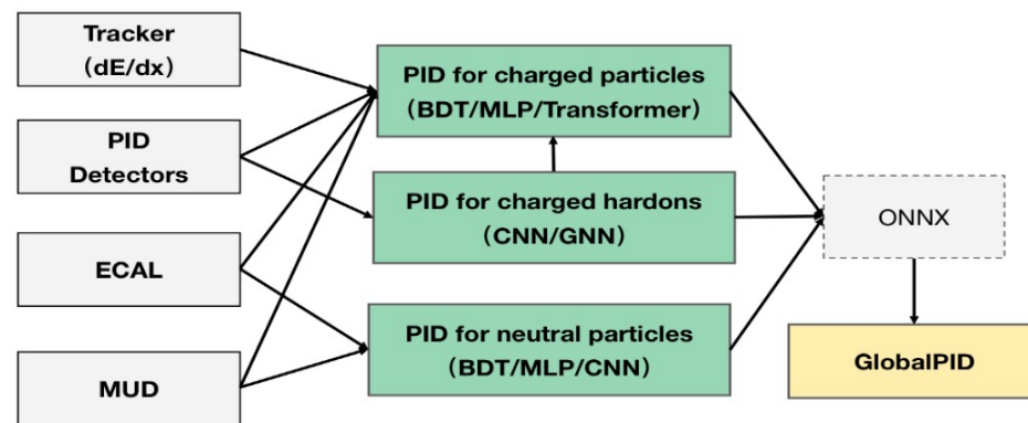
基于机器学习的STCF粒子识别算法
