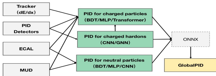
基于机器学习的STCF粒子识别算法
