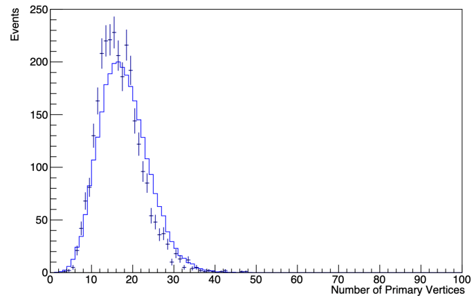
apply fourmu fit
