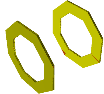
DD4hep_DiskTracker
