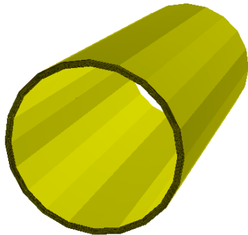
DD4hep_CylindricalBarrelCalorimeter
