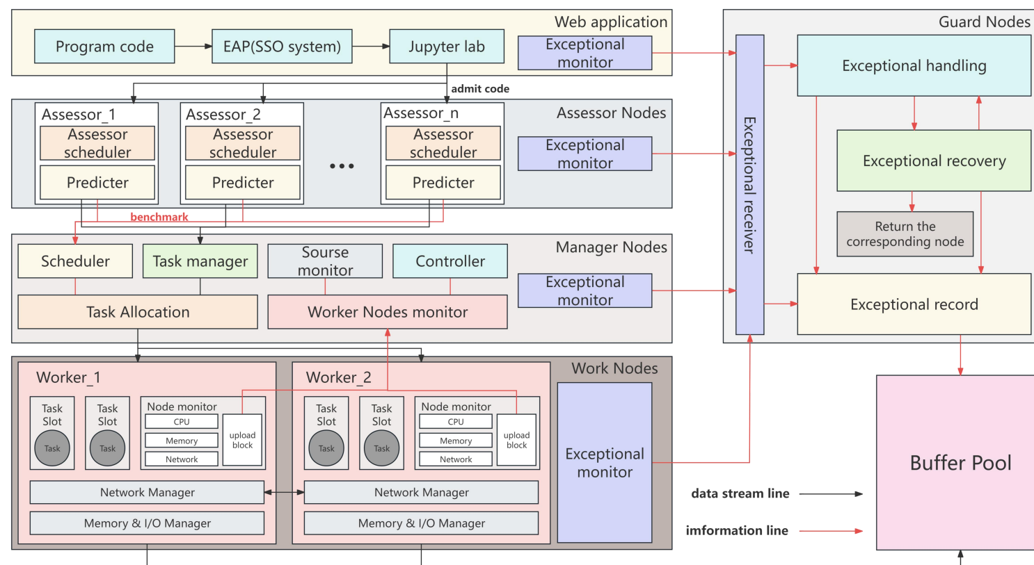
Schephy系统框图
