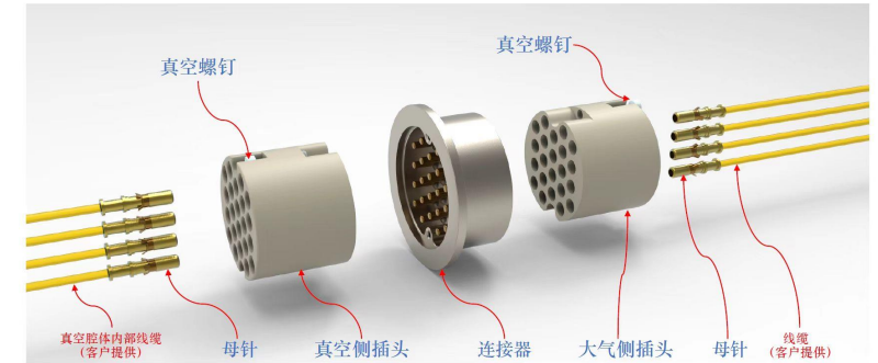
真空连接器 整体结构图
