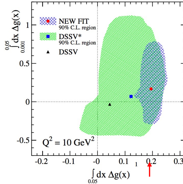
DSSV, PRL113 (2014) 012001
