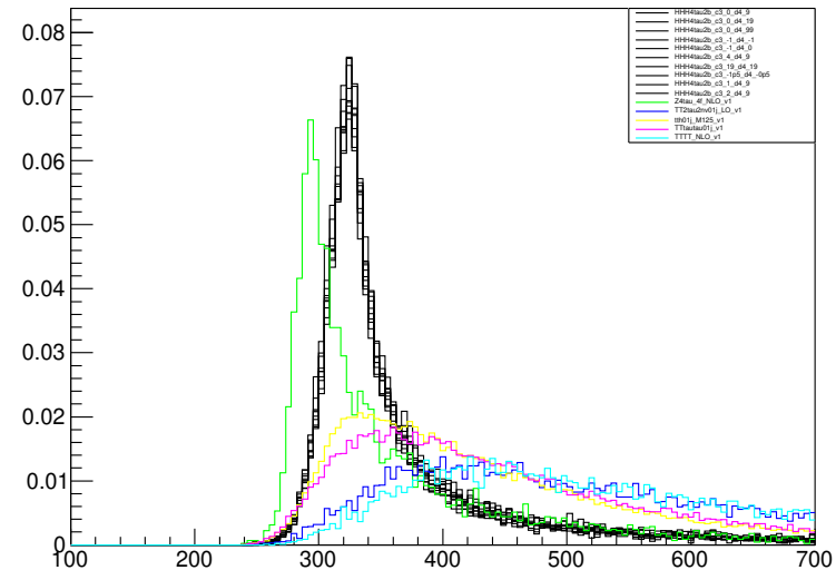
mT2_taupair1_2bj_200
