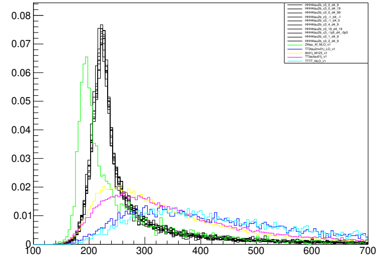
mT2_taupair1_2bj_200
