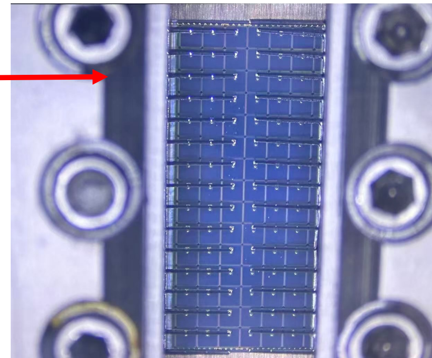
探针卡与LGAD芯片
