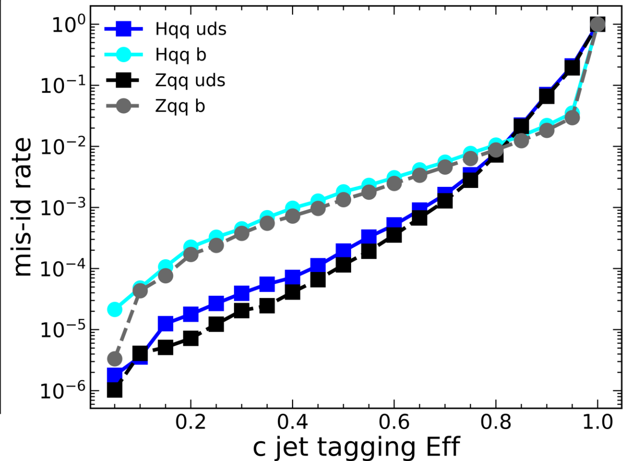
CEPC Ref-TDR
