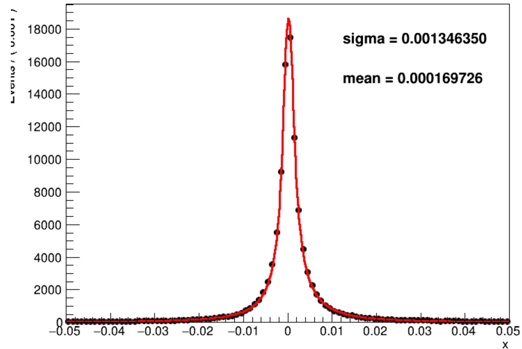
deltapt_sig
