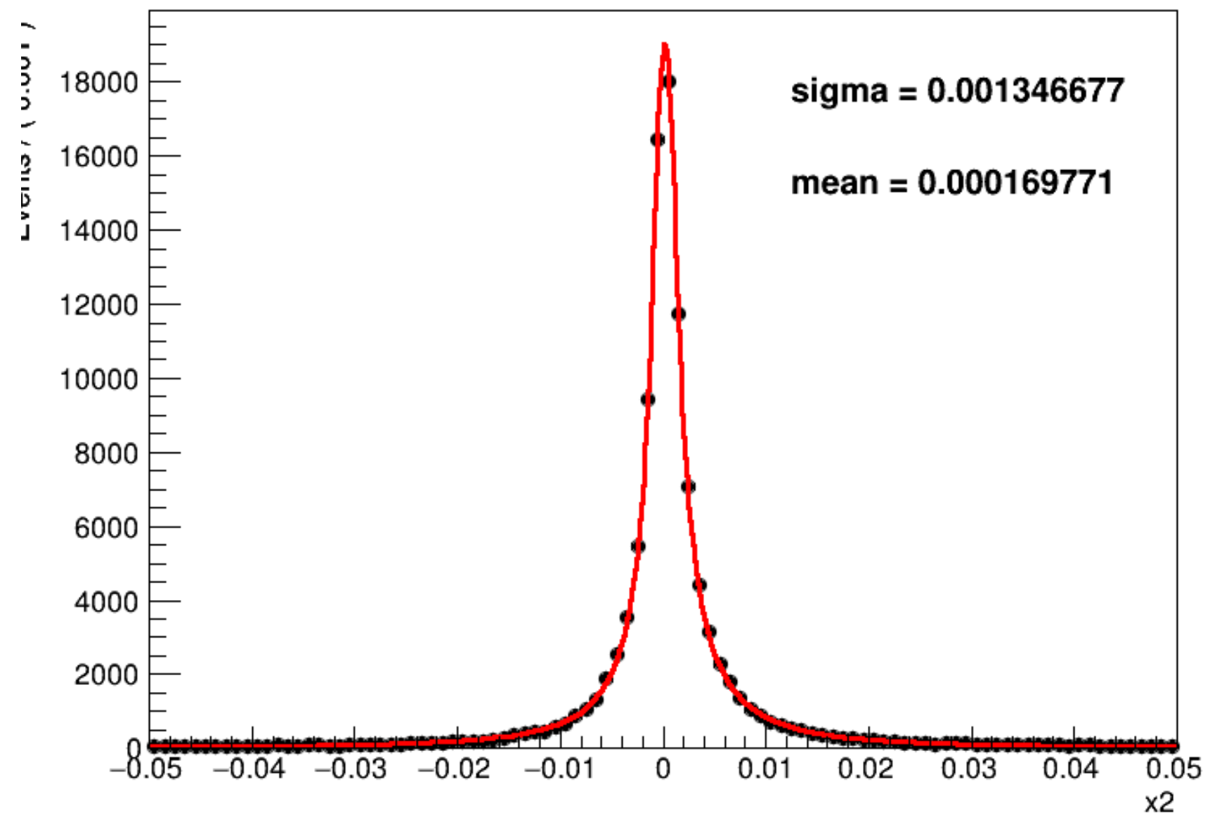
deltapt_sig
