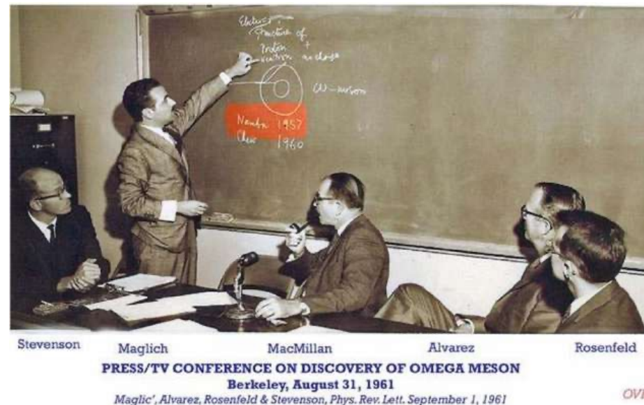
\omega 介子的发现
