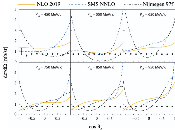
\Lambda p 弹性散射微分截面
