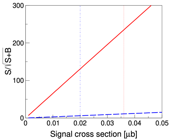
双重子态 d^* 显著度
