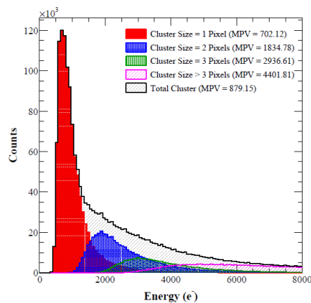
质子束流测试能谱
