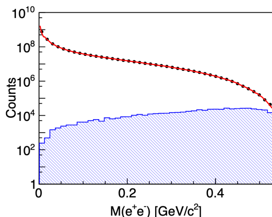
跃迁形状因子
