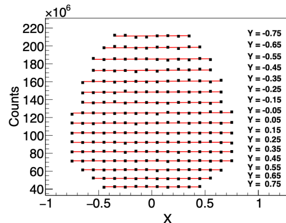
CP对称性检验
