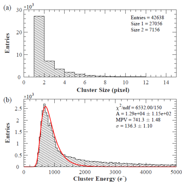
\beta 源测试结果
