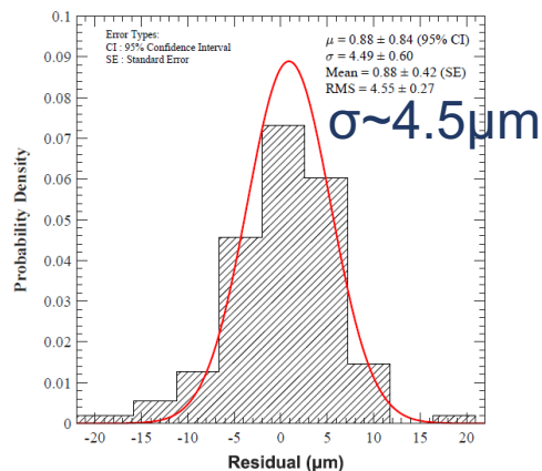
激光测试位置分辨
