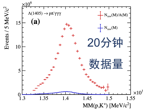
介子-重子分子态候选者 \Lambda(1405)
