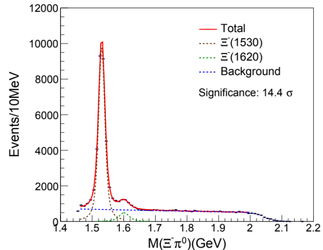
五夸克态候选者 \Xi(1620)^-
