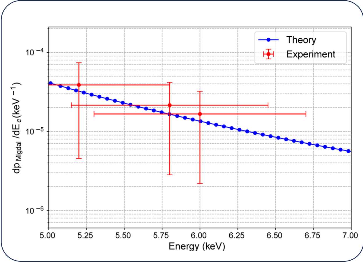
总跃迁几率
