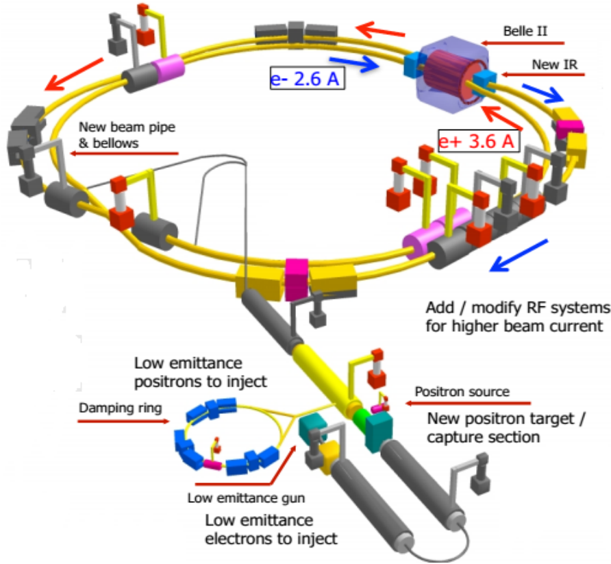
图 10.28: 日本KEK的Super-KEKB加速器示意图。
