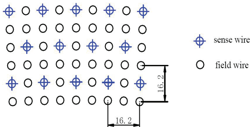
图 11.11: MDC单元结构示意图。
