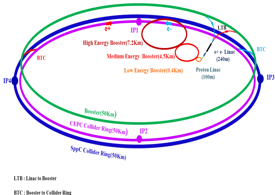
图 11.26: 正在讨论之中的中国正负电子对撞机-质子质子环形对撞机(CEPC-SPPC)的简单结构示意图。
