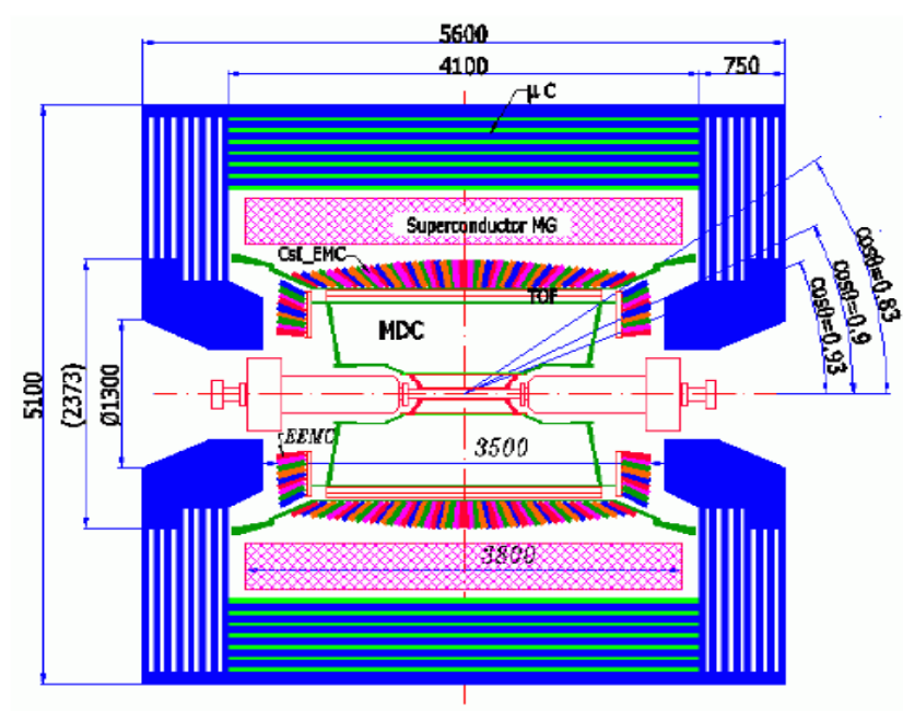
图 11.9: BESIII探测器总体结构侧视图
