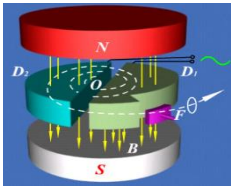
图 11.2: 回旋加速器示意图
