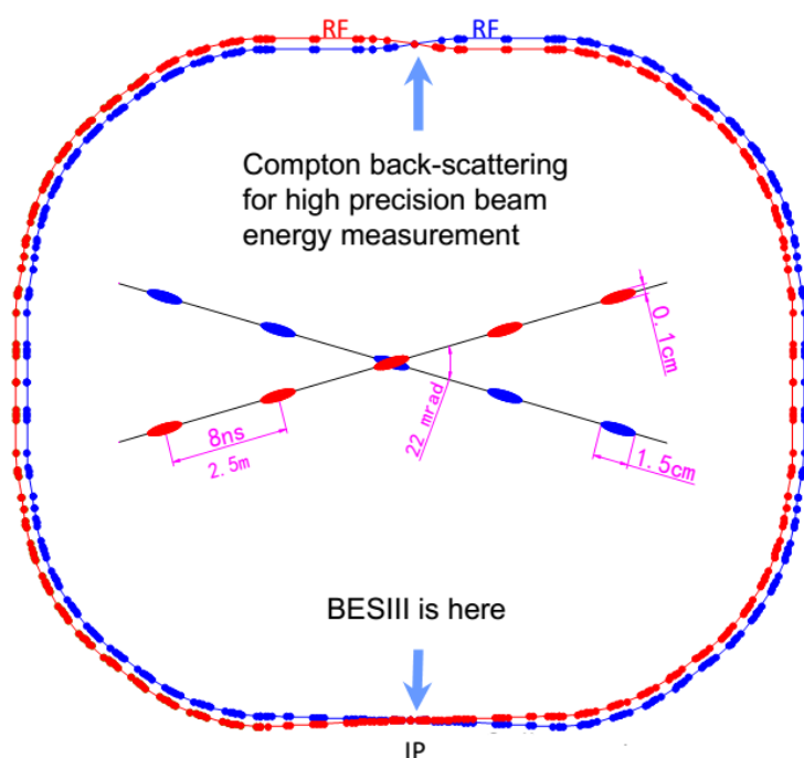
图 11.10: BEPC-II正负电子双环束流管的示意图。
