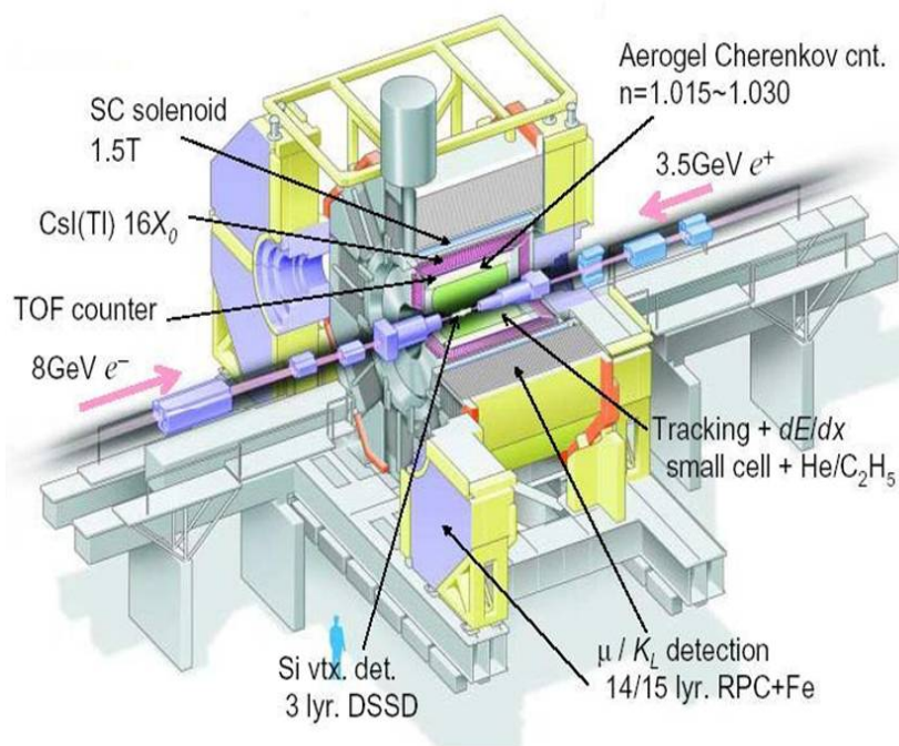
图 1.2: 在日本KEK B 工厂运行的Belle探测器。
