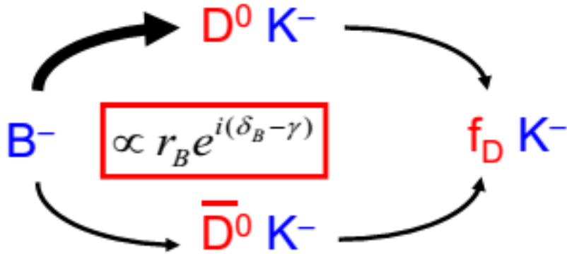
图 10.21: B^- \rightarrow D^0 K^-, \bar{D}^0 K^- 或者 B^- \rightarrow (D^{*0} K^{*-}, \bar{D}^{*0} K^{*-}) 衰变过程的费曼图。
