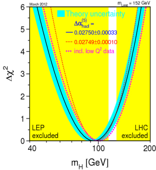
图 9.12: 2012年3月时, 根据标准模型理论研究和LEP, LHC等实验得到的对 M_H 的限制。黄色区域为被排除区域。
