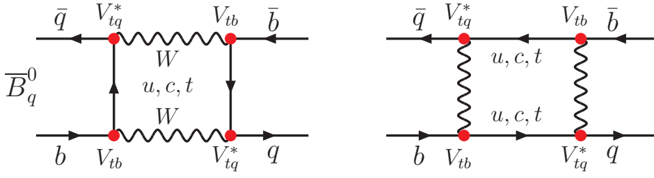
图 10.5: B_q^0 - \bar{B}_q^0 混合的箱图( q = (d, s) )。
