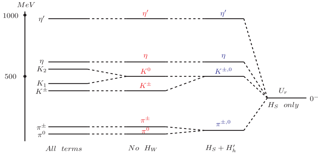
图 6.2: 0^- 介子超多重态结构。 H = H_S + H_W + H_{EM} + H'_h 。
