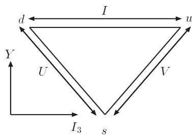
图 5.5: SU(3) 三重态包含 I , U , V 三个 SU(2) 二重态。
