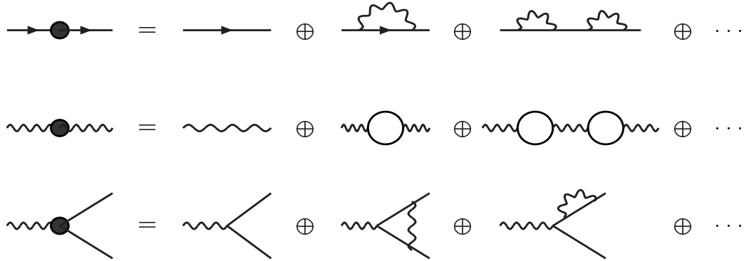
图 3.9: 量子电动力学(QED)中三种基本发散图形：电子自能图，真空极化图和顶角发散图。
