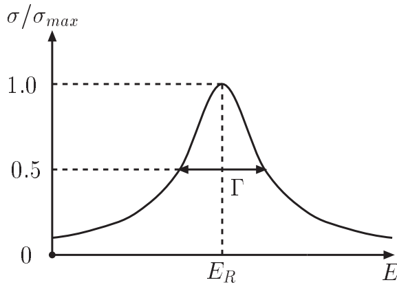
图 4.10: Breit-Wigner 共振曲线示意图。
