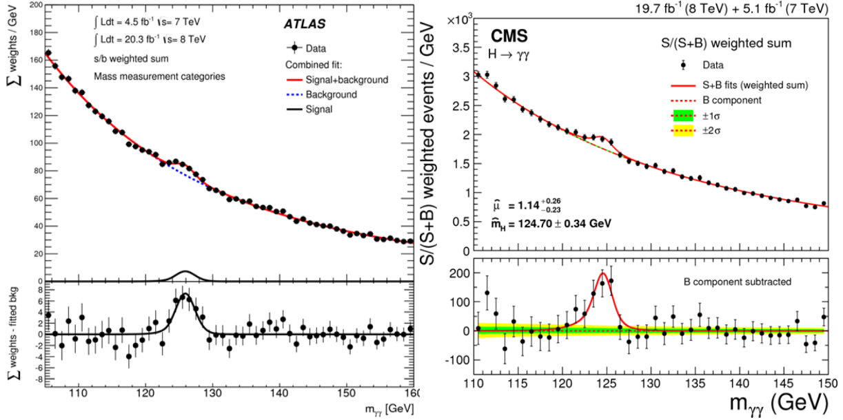
图 9.21: H \rightarrow \gamma\gamma 衰变道: ATLAS 和 CMS 实验组根据全部 RUN-1 数据分析得到的结果。
