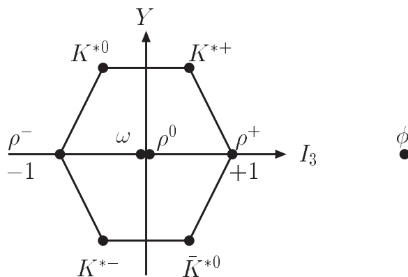
图 4.13: J^P = 1^- 的矢量介子八重态和单态。
