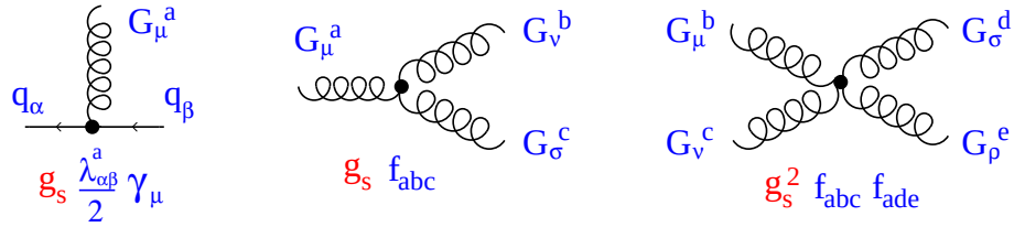
图 7.1: QCD拉氏量的相互作用顶角: 夸克胶子顶点, 三胶子顶点, 四胶子顶点。
