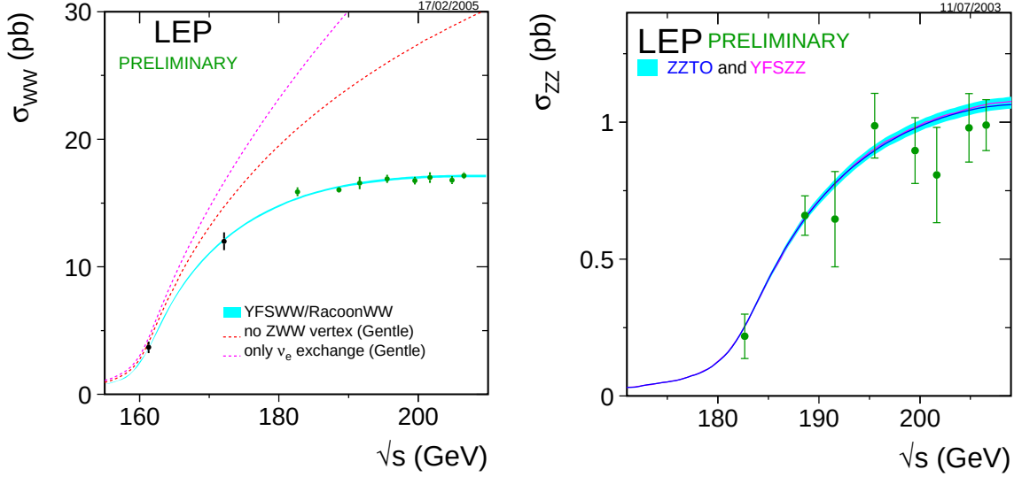
图 9.7: 产生截面 \sigma(e^+e^- \rightarrow W^+W^-) (左图)和 \sigma(e^+e^- \rightarrow Z^0Z^0) (右图)的质心能量依赖性, 不同理论预言值(实线和点线)和LEP实验测量结果[117, 123]。
