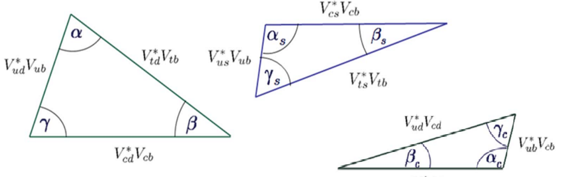
图 10.14: 根据CKM矩阵的么正性可以导出6个么正三角形。这是其中的3个么正三角形：分别对应 B_d^0 衰变， B_s 衰变和 D 介子衰变。
