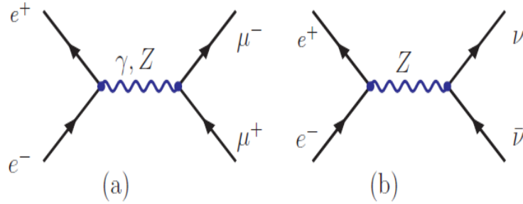
图 9.2: e^+e^- \rightarrow \mu^+\mu^- 和 e^+e^- \rightarrow \nu_\mu \bar{\nu}_\mu 过程的树图费曼图。
