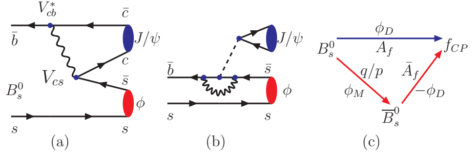
图 10.23: (a)与 \bar{b} \rightarrow c\bar{c}s\bar{s} 衰变对应的树图贡献; (b)色单态(虚线)企鹅图贡献(内线夸克为 (u, c, t) ); (c)示意图: B_s^0 \rightarrow f_{CP} 的直接衰变和 B_s^0 \rightarrow \bar{B}_s^0 \rightarrow f_{CP} 的衰变。
