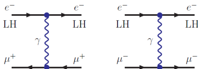
图 3.11: 电子和 \mu 子散射 e^-\mu^+ \rightarrow e^-\mu^+ , e^-\mu^- \rightarrow e^-\mu^- 的领头阶费曼图。
