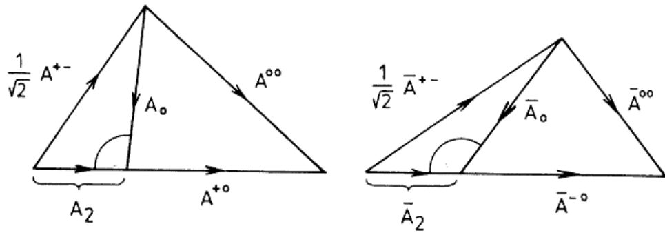
图 10.20: B \rightarrow \pi\pi 的三个衰变振幅之间的同位旋三角形关系[170]。
