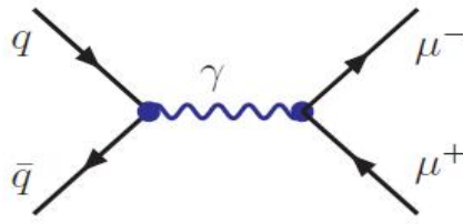
图 3.12: 强子碰撞中“Drell-Yan”轻子对产生过程的领头阶费曼图。
