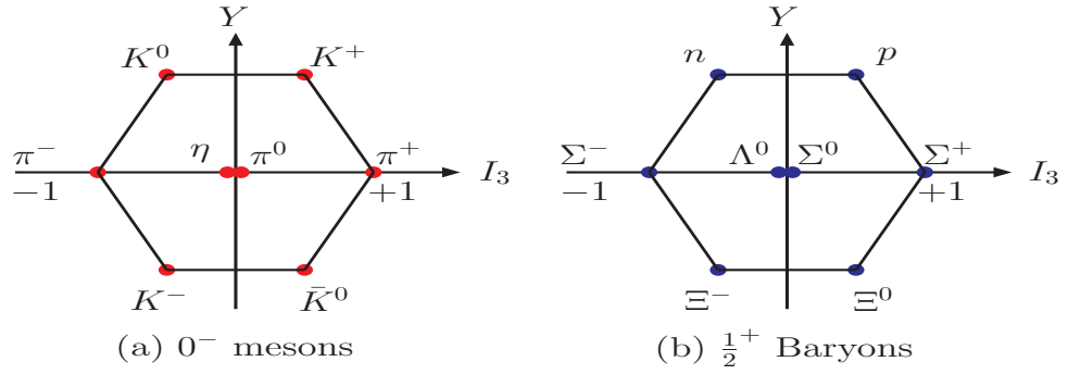
图 4.7: (a) SU (3) 八重态的 0^- 介子, (b) \frac{1}{2}^+ 的重子八重态。
