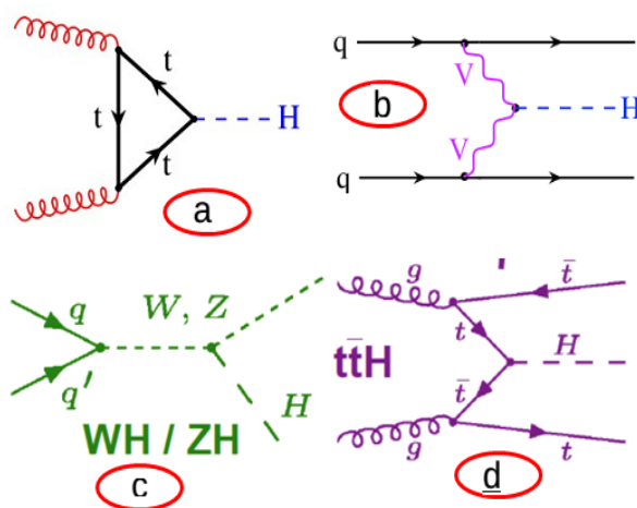
图 9.13: 在LHC实验中Higgs玻色子主要产生过程的费曼图:(a) 胶子聚合道, gg \rightarrow H ; (b) 规范玻色子聚合道, WW/ZZ \rightarrow H ; (c) WH/ZH 伴随产生道, qq' \rightarrow WH, ZH ; (d) gg \rightarrow t\bar{t}H 产生道。
