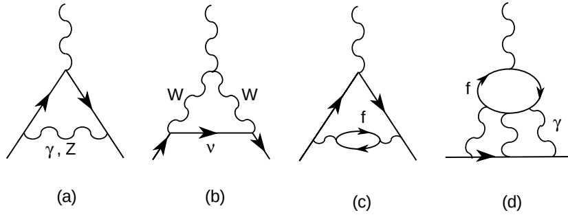
图 3.7: 对轻子反常磁矩有贡献的典型低阶费曼图。
