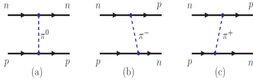
图 4.1: 核力的汤川模型: 直接作用(a) 和交换作用(b,c)。
