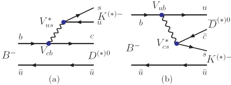
图 10.21: B^- \rightarrow D^0 K^-, \bar{D}^0 K^- 或者 B^- \rightarrow (D^{*0} K^{*-}, \bar{D}^{*0} K^{*-}) 衰变过程的费曼图。
