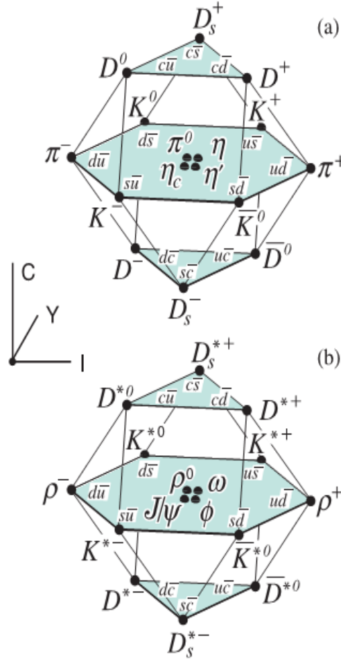
图 6.18: 由轻夸克( u, d, s )和 c 夸克构成的16重态 SU(4) 权图: (a) 赝标量介子; (b) 矢量介子。三个坐标轴分别表示粒子的同位旋“ I ”, 超荷“ Y ”与粲数“ C ”。
