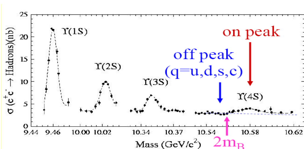
图 6.15: \Upsilon(NS) 共振态( N = 1, 2, 3, 4 ).
