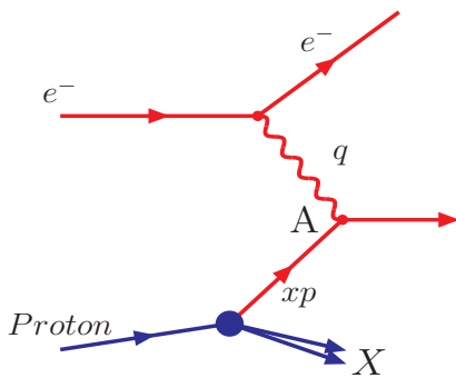
图 7.9: 在部分子模型中，入射的电子与质子内部（近似自由）的部分子发生散射。
