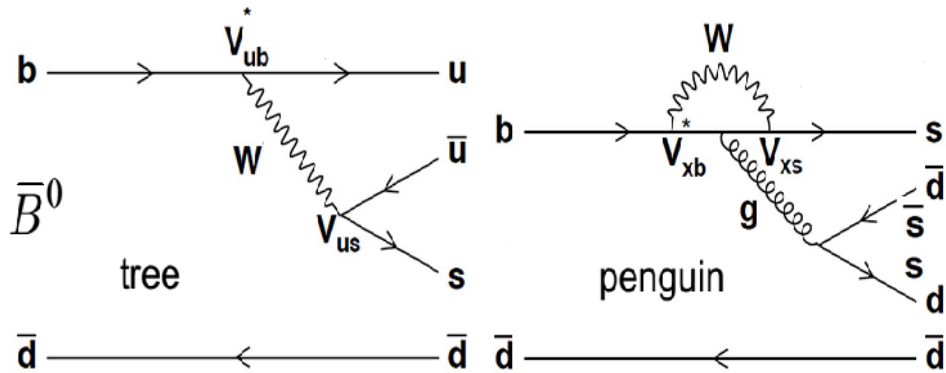
图 10.16: 与 b \rightarrow q\bar{q}s 相关联的 B 介子两体强子衰变过程。左侧的树图过程被双重压低：色压低( 1/N_c )和CKM压低( \lambda^2 )，右侧的企鹅图贡献起主要作用。
