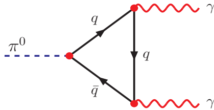
图 6.6: 通过夸克三角图进行的 \pi^0 \rightarrow 2\gamma 衰变。
