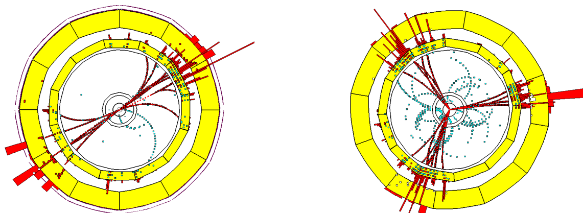
图 7.2: 在LEP e^+e^- 对撞机上ALEPH实验组观察到的 Z^0 玻色子的强子衰变过程的2-喷注和三喷注事例： Z^0 \rightarrow q\bar{q} 和 Z^0 \rightarrow q\bar{q}G 。
