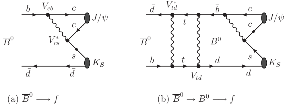
图 10.15: B_d^0 \rightarrow J/\psi K_S^0 衰变过程费曼图。(a) \bar{B}^0 \rightarrow J/\psi K_S 树图；(b) \bar{B}^0 \rightarrow B^0 \rightarrow J/\psi K_S 混合-衰变费曼图。
