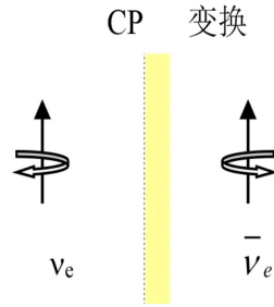
图 5.4: 中微子和反中微子之间通过CP变换相联系。
