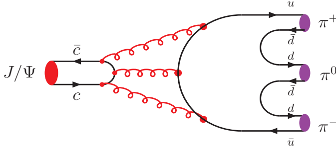
图 6.14: 通过3胶子交换实现的 J/\Psi \rightarrow 3\pi 湮灭道产生过程。
