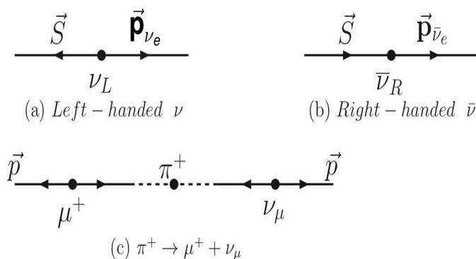
图 3.4: \pi^+ \rightarrow \mu^+ + \nu_\mu 衰变中在 \pi^+ 的静止坐标系中观测到的 \mu^+ 和 \nu_\mu 的螺旋度。
