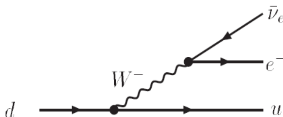
图 3.3: 原子核 \beta 衰变的夸克层次费曼图。
