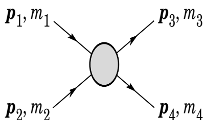
图 2.8: 2 \rightarrow 2 散射过程的示意图。
