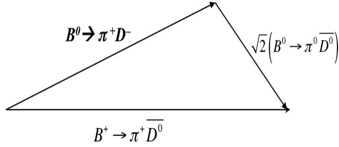
图 4.4: 三个 B \rightarrow D\pi 衰变道的衰变振幅在复平面上形成的三角形同位旋关系示意图。
