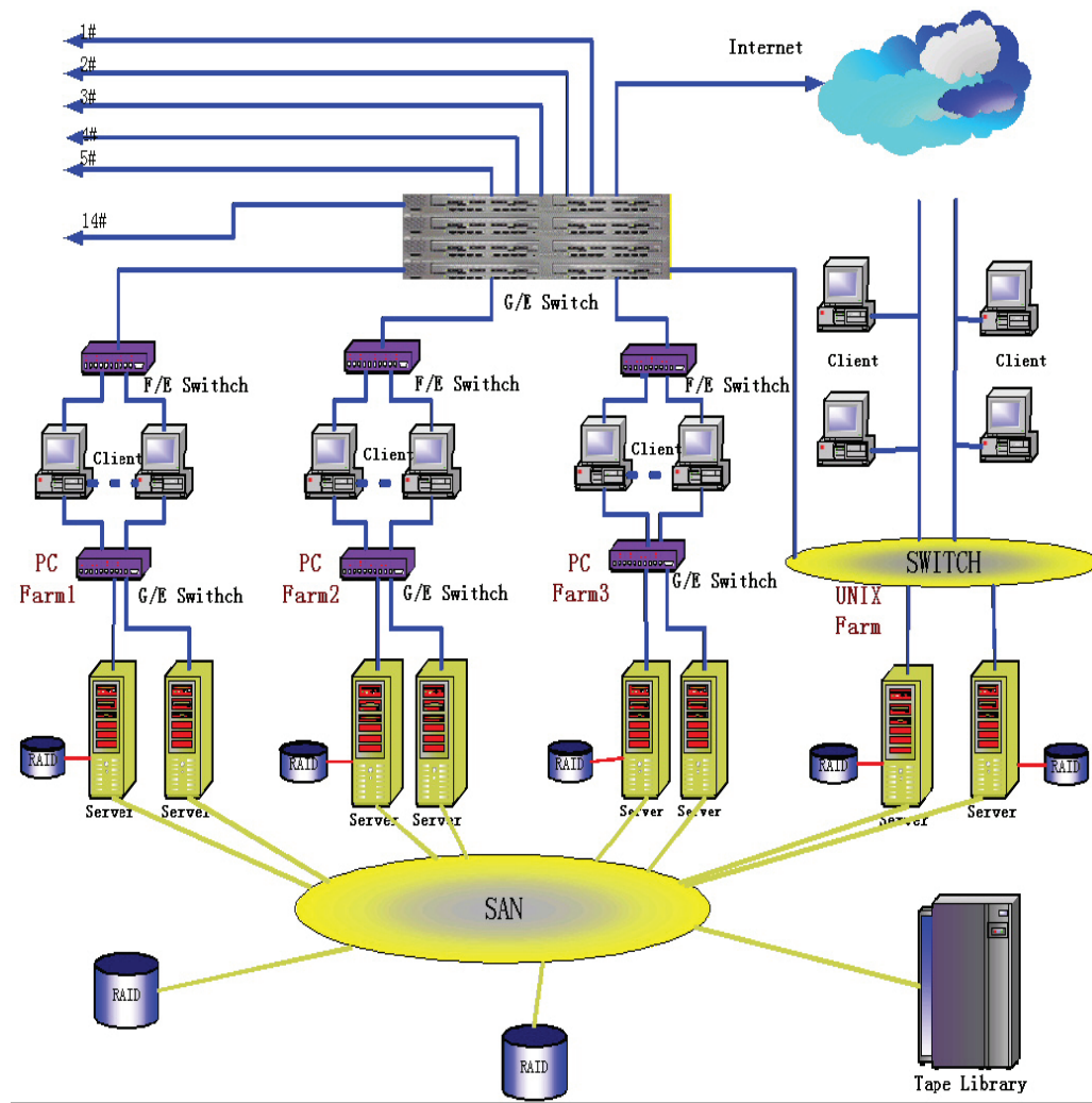
图 11.19: BESIII数据处理系统结构示意图
