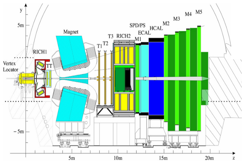
图 1.4: LHC-b 专用探测器。
