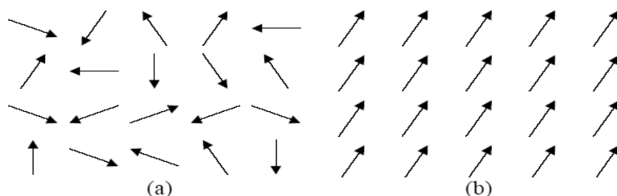
图 8.2: 顺磁相(a)和铁磁相(b)的自旋方向示意图。
