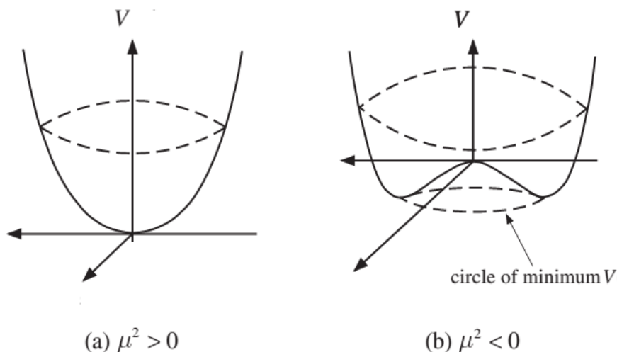
图 8.3: 与严格对称性对应的真空态(a): \mu^2 > 0 。与破缺对称性对应的真空态(b): \mu^2 < 0 。
