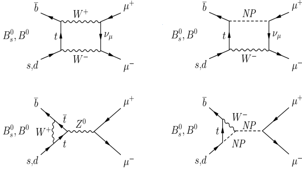
图 10.10: 在标准模型(左侧两个费曼图)和新物理模型(右侧两个费曼图)框架下对 B_{s,d}^0 \rightarrow \mu^+ \mu^- 纯轻子衰变过程有贡献的单圈费曼图。
