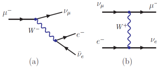
图 9.1: 描写 \mu^- \rightarrow e^- \bar{\nu}_e \nu_\mu 和 \nu_\mu e^- \rightarrow \mu^- \nu_e 过程的树图费曼图。
