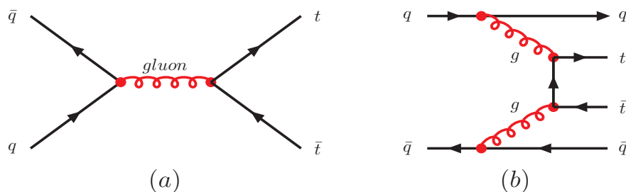
图 6.16: 在Tevatron p\bar{p} 对撞机上主要的 t\bar{t} 对产生费曼图。
