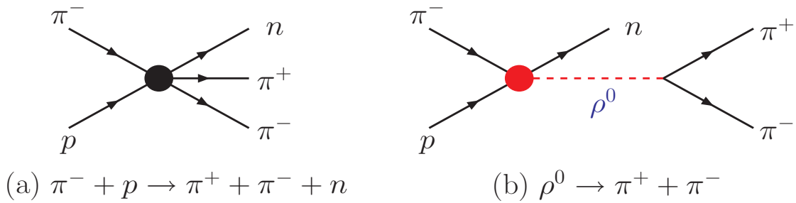
图 2.6: (a) 二体碰撞直接产生三体末态的示意图 \pi^- + p \rightarrow \pi^+ + \pi^- + n ; (b) 二体碰撞先产生二体末态 \pi^- + p \rightarrow \rho^0 + n , 然后其中的 \rho^0 介子衰变 \rho^0 \rightarrow \pi^+ + \pi^- 。
