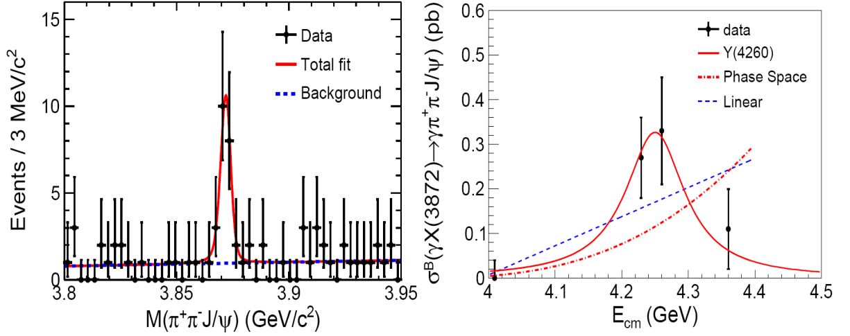
图 11.22: BES-III合作组对 M(\pi^+\pi^-J/\Psi) 不变质量分布的拟合结果(左图), 对产生率 \sigma^B(e^+e^- \rightarrow \gamma X(3872))\mathcal{B}(X(3872) \rightarrow \pi^+\pi^-J/\Psi) 的拟合结果(右图)[194]。
