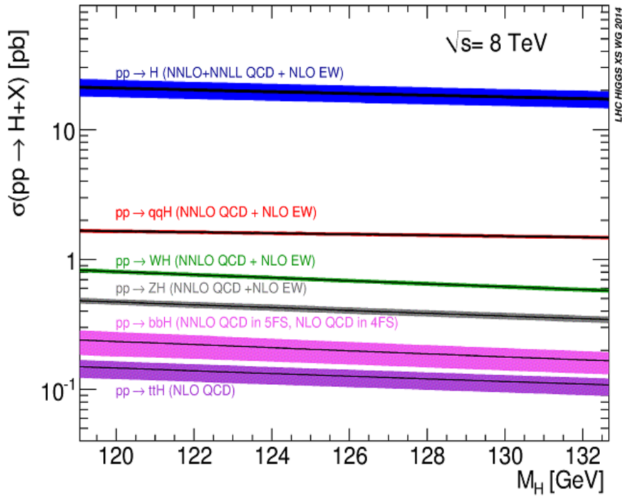
图 9.14: 质心系能量为 \sqrt{S} = 8\text{TeV} , 118 \leq m_H \leq 133\text{ GeV} 时, 对产生截面 \sigma(pp \rightarrow H + X)(\text{pb}) 的标准模型理论预言。在图中给出了 ggH 等各个主要产生道的产生截面, 以及目前理论计算达到的精度。
