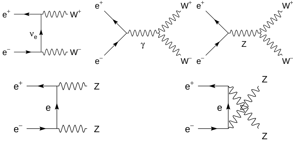
图 9.6: e^+e^- \rightarrow W^+W^- 和 e^+e^- \rightarrow ZZ 规范玻色子对产生过程的树图费曼图。
