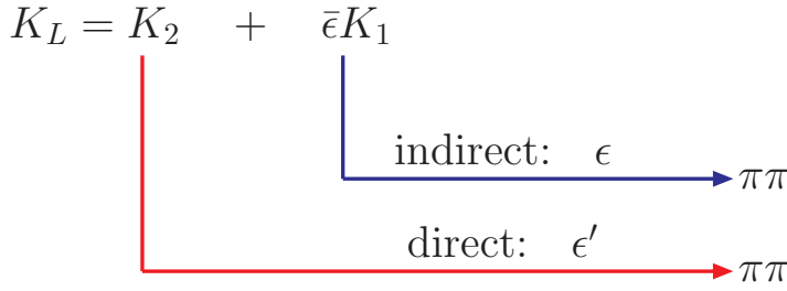
图 10.3: K_L \rightarrow \pi\pi 衰变过程中的直接和间接CP破坏示意图。
