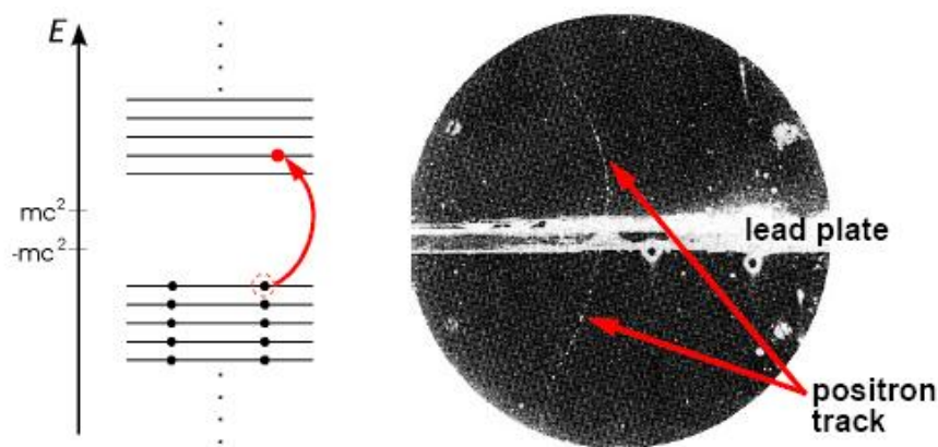
图 3.15: 在狄拉克真空中的电子和正电子(左图); 在Wilson云室中正电子轨迹照片(右图)。
