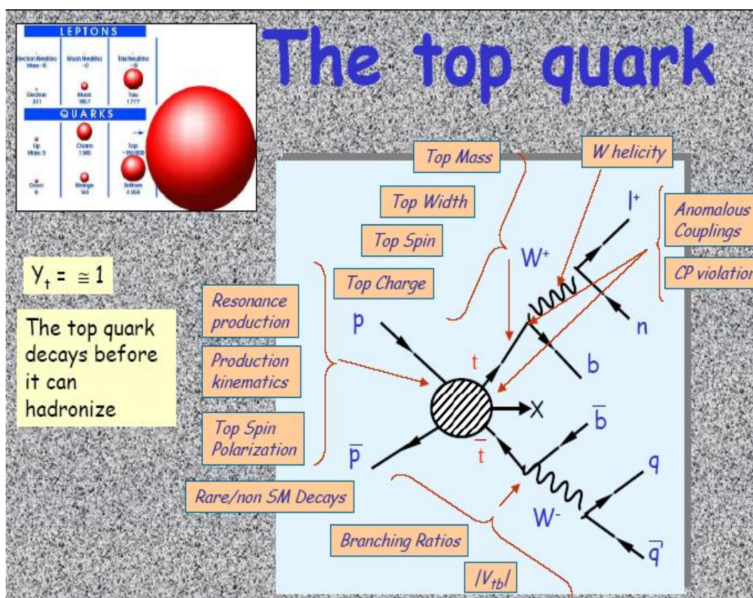
图 6.17: Top 夸克的产生和衰变的费曼图-示意图[78]。
