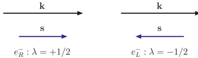
图 1.6: 电子的螺旋度-左旋 (L) 和右旋 (R) 定义： e_L^- 和 e_R^- 。
