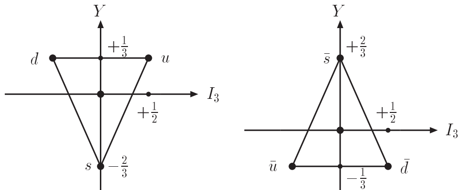
图 6.5: SU(3) 的基础表示 “3” 和复共轭表示 “ \bar{3} ” : 3 = (u, d, s) , \bar{3} = (\bar{u}, \bar{d}, \bar{s}) 。
