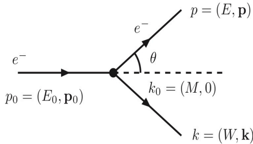
图 7.4: 在靶粒子静止系， eN 散射四动量变化。
