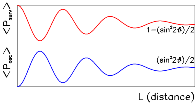
图 3.6: 对能量分布做平均后的中微子振荡几率 \mathcal{P}_{osc} 和再现几率 \mathcal{P}_{\alpha\alpha} = 1 - \mathcal{P}_{osc} 随距离 L 的变化。
