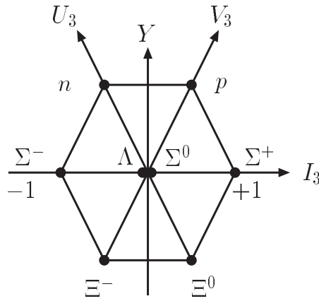
图 6.3: \frac{1}{2}^+ 重子八重态。强子的么正对称性，U 旋和 V 旋。
