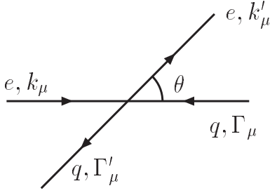
图 7.13: 在质心系中的 e + q \rightarrow e + q 散射过程。
