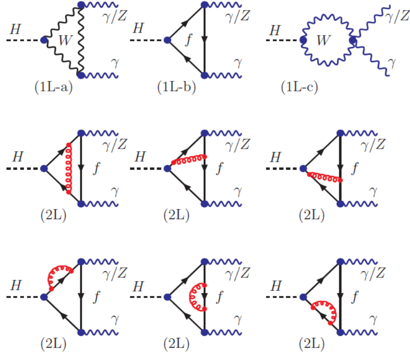
图 9.20: 在标准模型下, H \rightarrow \gamma\gamma ( H \rightarrow Z\gamma ) 的领头阶单圈费曼图(第一行), 对单圈夸克费曼图的双圈QCD修正的费曼图(第二、第三行)。在双圈(单圈图)中的 f 表示带电的夸克(轻子和夸克)。
