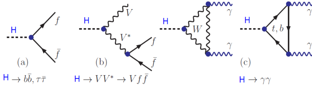
图 9.15: LHC实验上观测到的Higgs玻色子的主要衰变道的最低阶费曼图: (a) H \rightarrow f\bar{f} ( f = l^-, q \neq t ); (b) H \rightarrow VV^* \rightarrow V f \bar{f} ; (c) H \rightarrow 2\gamma 。
