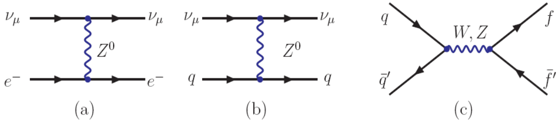
图 8.1: (a,b) 实验上发现的中性弱流的领头阶费曼图。(c)由交换带电和中性矢量玻色子 W^\pm, Z^0 引起的 2 \rightarrow 2 s-道产生过程的领头阶费曼图。
