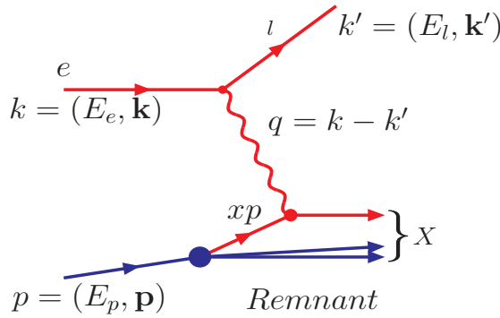
图 7.11: e + p \rightarrow l + X 。 l = e 时为中性流过程； l = \nu_e 时为带电流过程。
