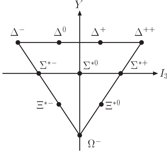
图 4.11: J^P = \frac{3}{2}^+ 的重子十重态。
