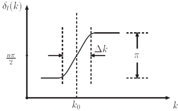
图 4.8: 在 k_0 处有共振态时, \delta_l(k) 随 k 变化的关系。
