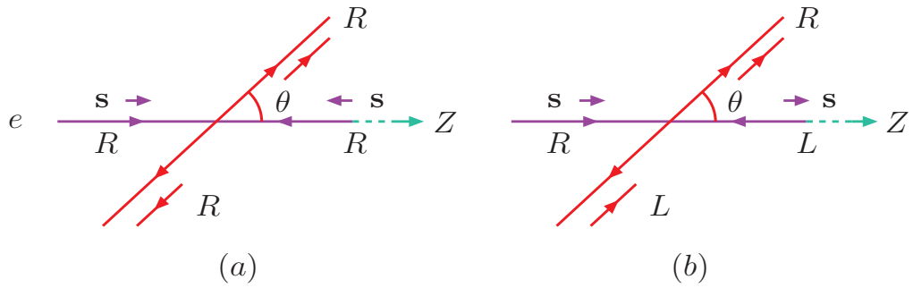
图 7.14: 在质心系对 e + q \rightarrow e + q 散射过程的螺旋度分析: (a) RR \rightarrow RR ; (b) RL \rightarrow RL 。
