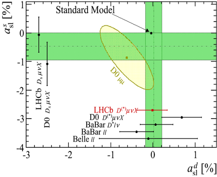
图 10.7: D0实验组、B介子工厂实验和LHCb实验组对参数 a_{SL}^d (横坐标)和 a_{SL}^s (纵坐标)的实验测量结果。
