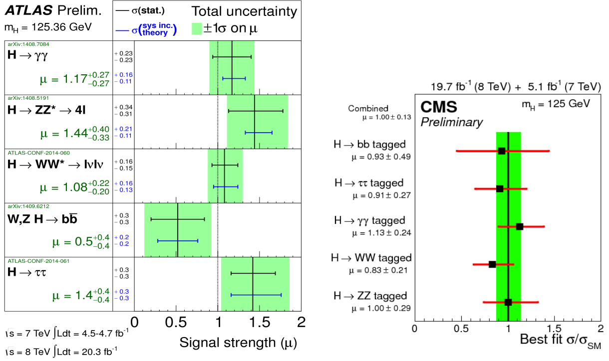
图 9.18: 基于全部RUN-1数据, ATLAS和CMS实验组对Higgs玻色子的5个主要衰变道的信号强度 \mu = \sigma_{\text{meas}}/\sigma_{\text{SM}} 的实验测量结果。
