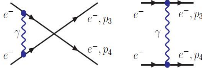
图 3.14: Moeller散射过程 e^-e^- \rightarrow e^-e^- 的领头阶费曼图。
