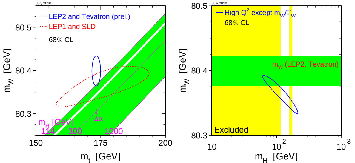
图 9.3: 左图表示根据LEP-I和SLD实验数据得到的对 m_W - m_t 取值范围的间接限制(点线Contour-plot), 根据LEP-II和Tevatron实验数据得到的对 m_W - m_t 取值范围的限制(实线Contour-plot)。在这两种情况下的Contour-plot的置信度均为68%。右图表示根据标准模型和相关实验数据(大- Q^2 数据, 但不包含对 m_W 和 \Gamma_W 的直接实验测量数据)对 m_W - m_H 取值区域给出的限制
