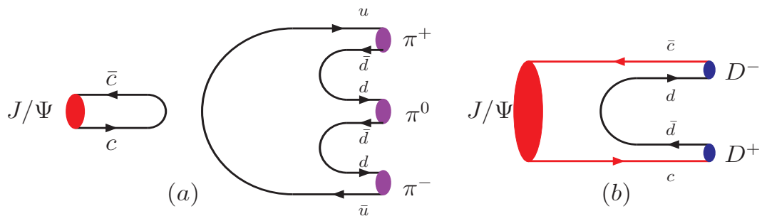
图 6.13: J/\Psi 介子的可能衰变道。(a) 被强烈压低的湮灭衰变道，图中的半椭圆表示可能的高阶QCD和电弱修正，(b) 被OZI 规则允许但相空间不允许的可能衰变道。
