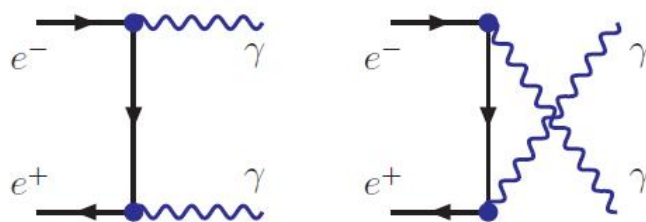
图 3.10: 正负电子湮灭到两个光子 e^+e^- \rightarrow \gamma\gamma 的领头阶费曼图。
