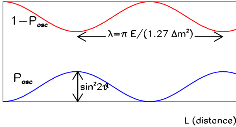
图 3.5: 振荡几率 \mathcal{P}_{osc} 和再现几率 \mathcal{P}_{\alpha\alpha} = 1 - \mathcal{P}_{osc} 随距离 L 的变化。
