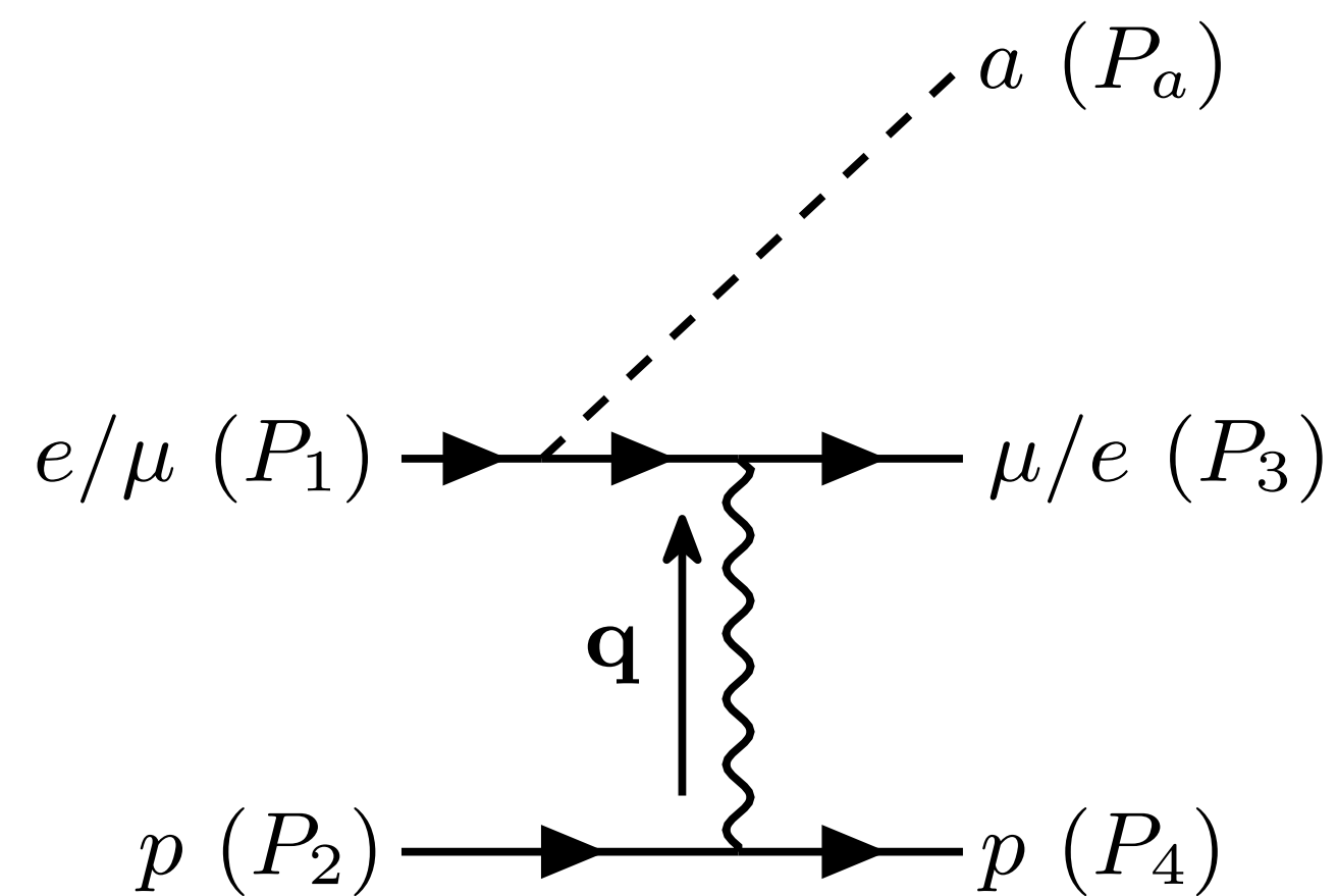
bremsstrahlung
