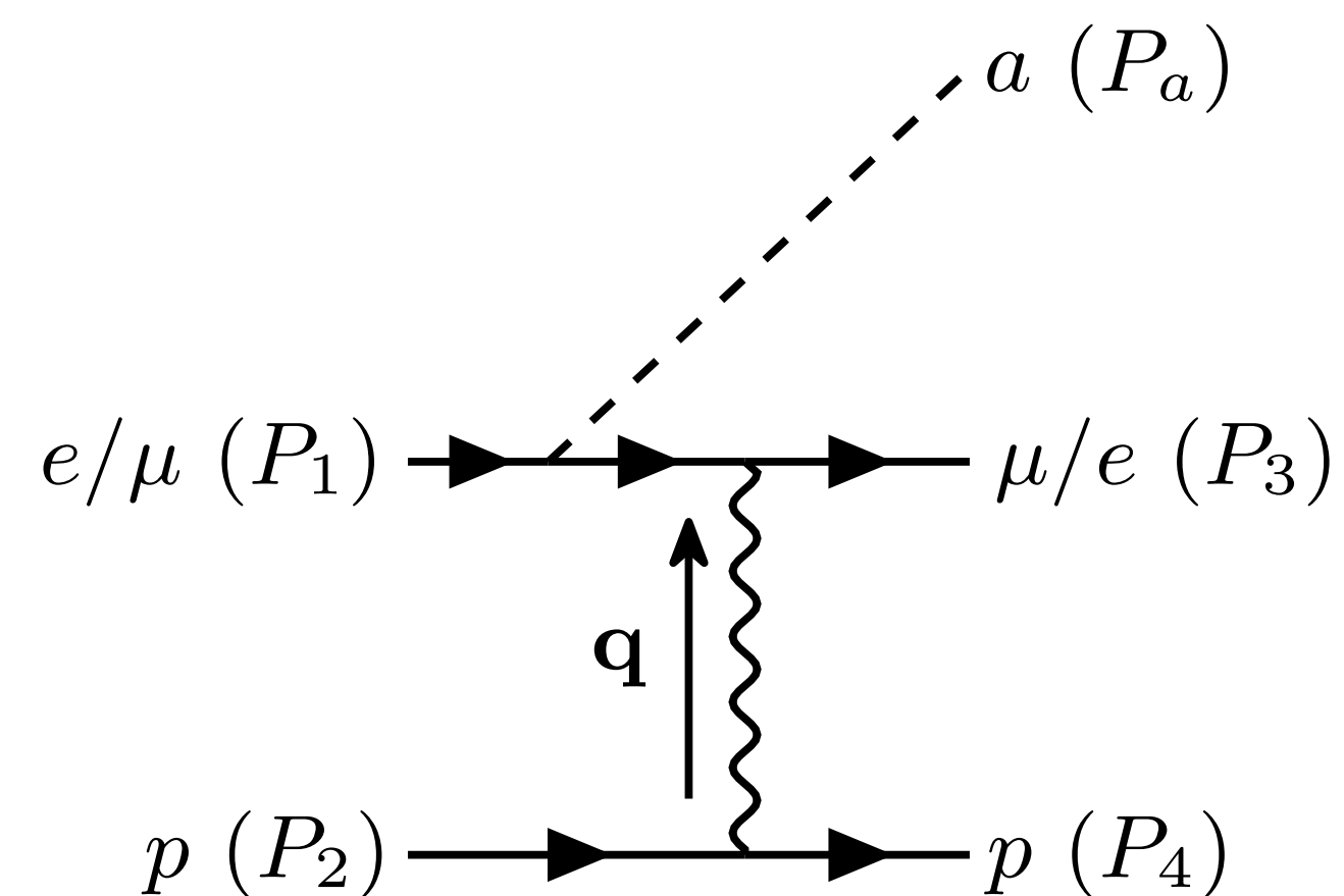
bremsstrahlung
