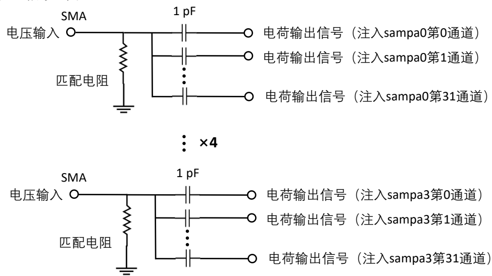
注入板原理图
