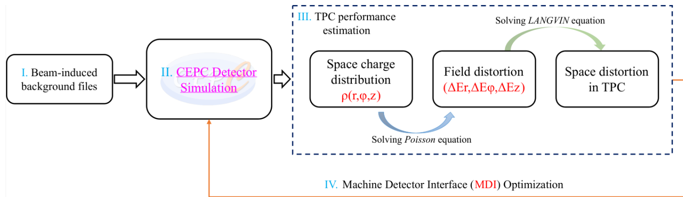
TPC束流本底模拟流程
