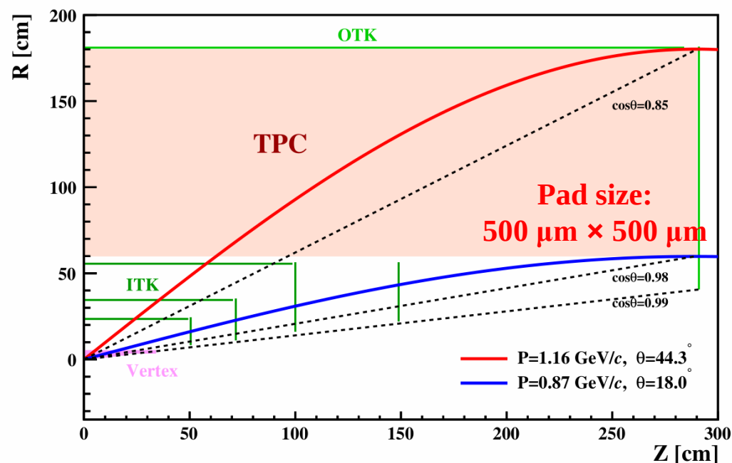
CEPC 径迹系统 (Tracker system) R-Z平面布局
