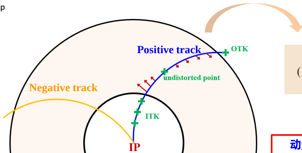
空间电荷效应带来的测量点畸变示意图
