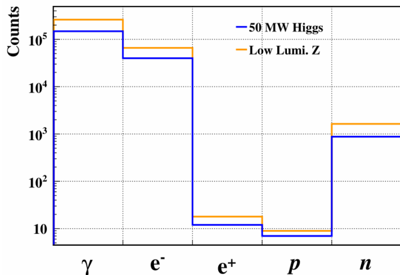
单位时间内进入TPC束流本底粒子种类分布
