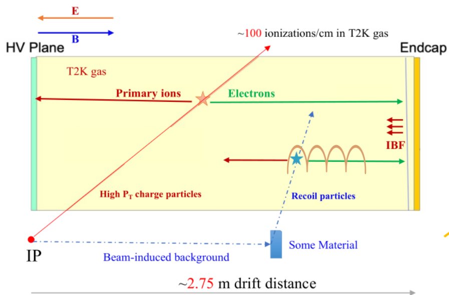
TPC中空间电荷来源示意图
