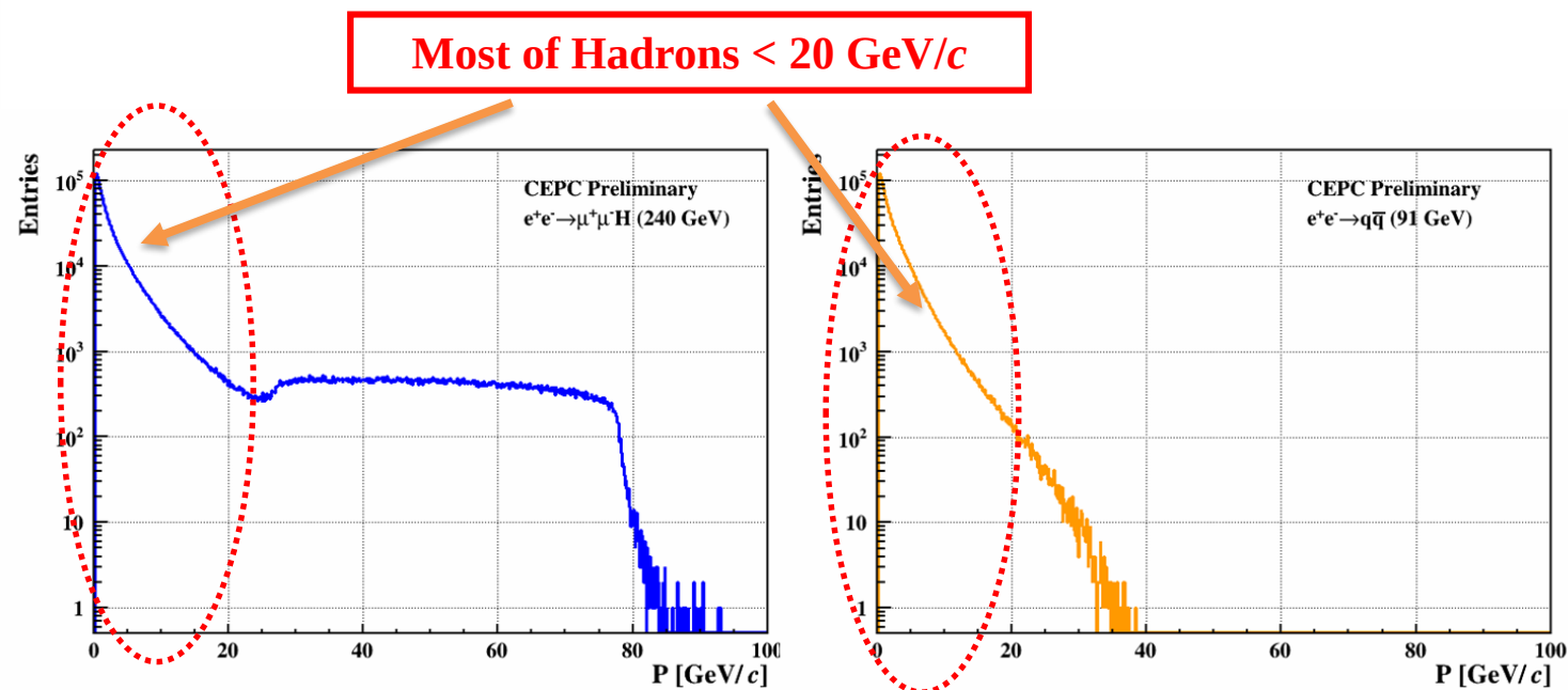
CEPC 不同物理过程末态带电粒子动量分布, (左) e^+e^- \rightarrow \mu^+\mu^-H , (右) e^+e^- \rightarrow q\bar{q}
