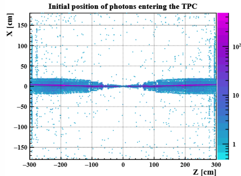
低能光子产生区域
