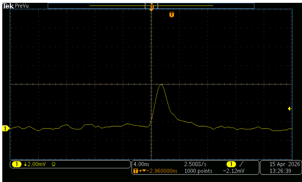
暗计数测试, 平均半高宽约1.3 ns
