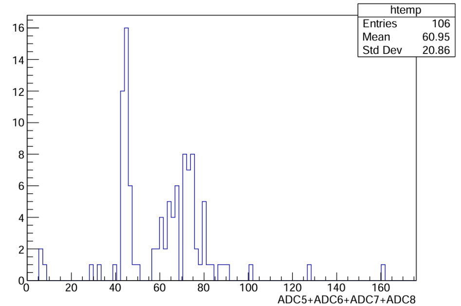
ADC5+ADC6+ADC7+ADC8
