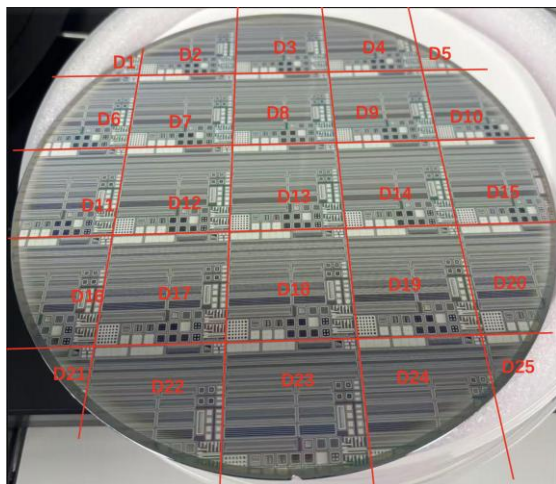
Latest AC-LGAD Wafer
