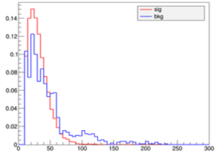
Antimuon PT
