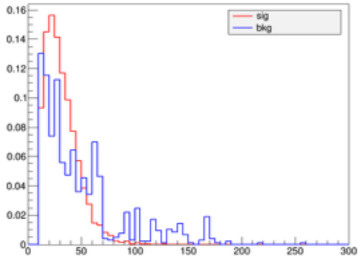
Positron PT
