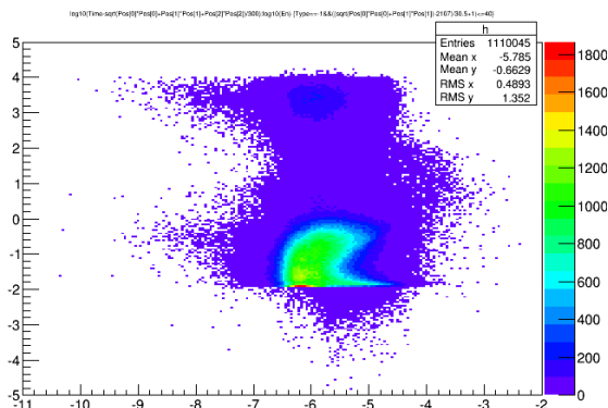
总1110045
