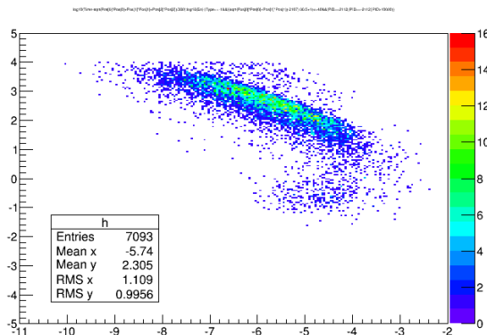
中子(7093,6.4%)
