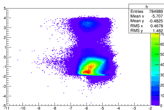
电子光子784949,70.7%
