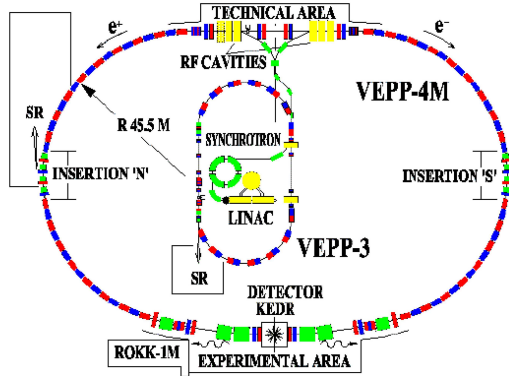
Fig. 2. VEPP-4M collider.
