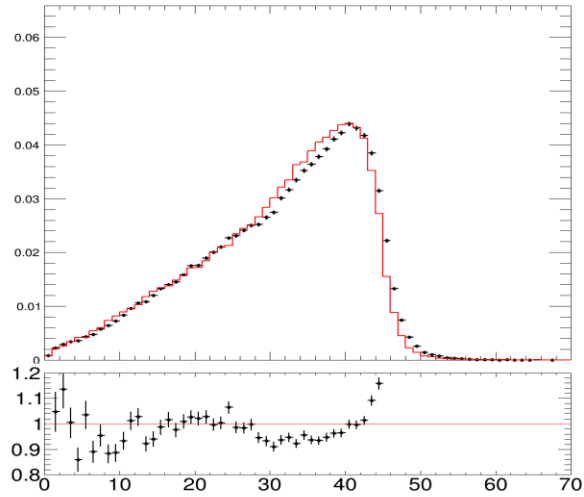
Jet_pt
