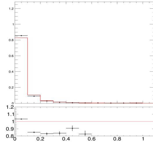
Jet_prob
