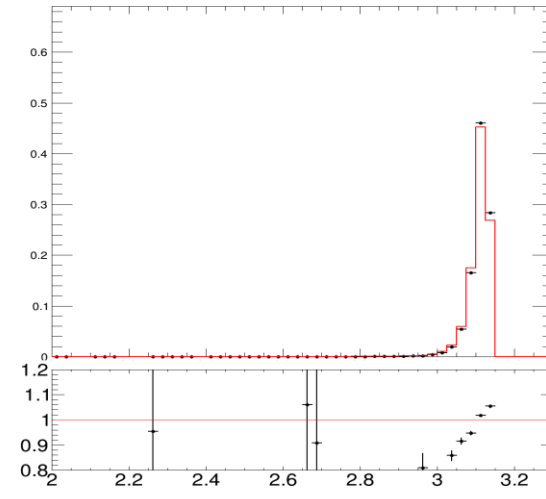
Angle_jet1vsjet2
