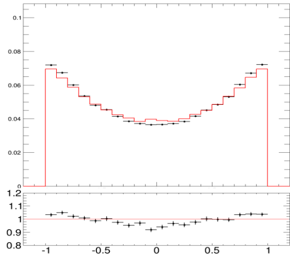
cosθ
