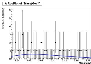
(b) background PDF
