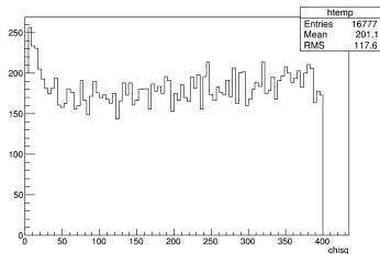
(d) \chi^2_{4C} of background events
