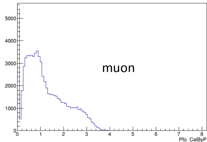
CalByP: (e_{\text{cale}} + h_{\text{cale}}) / p
