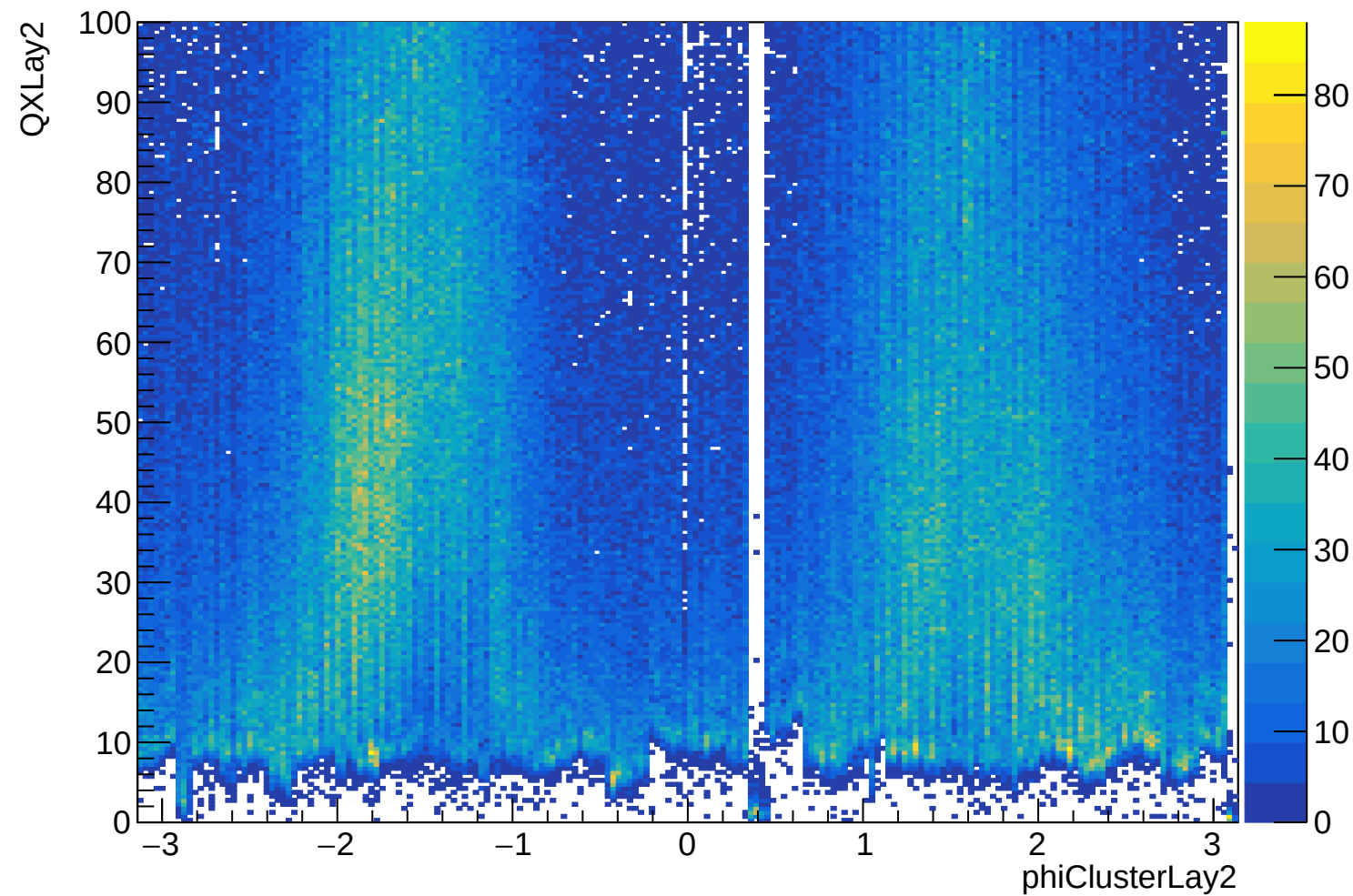
QXLayer2:phiClusterLayer2 {nXStripsLayer2>1}
