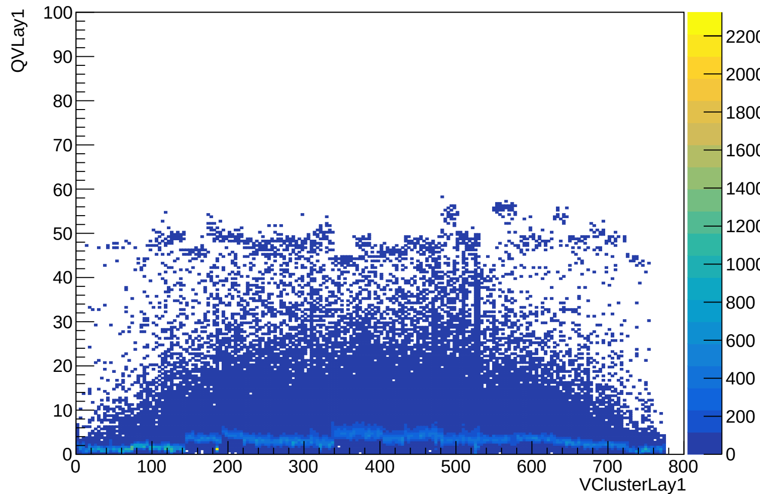
QVLay1:VClusterLay1 {nVStripsLay1==1}
