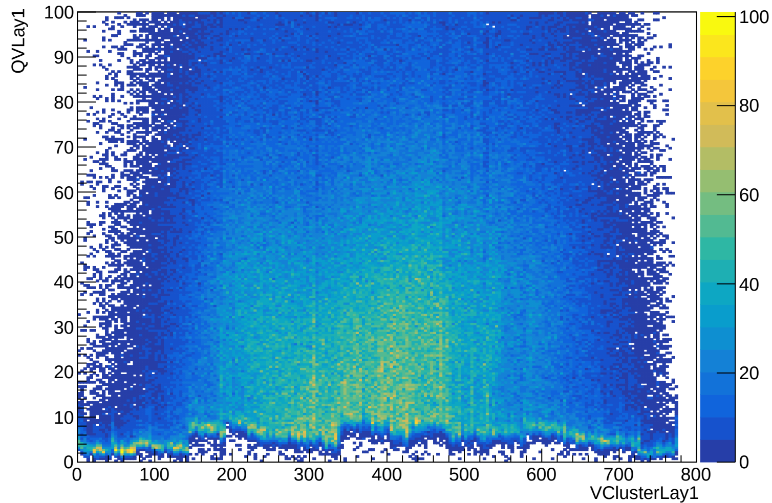
QVLay1:VClusterLay1 {nVStripsLay1>1}
