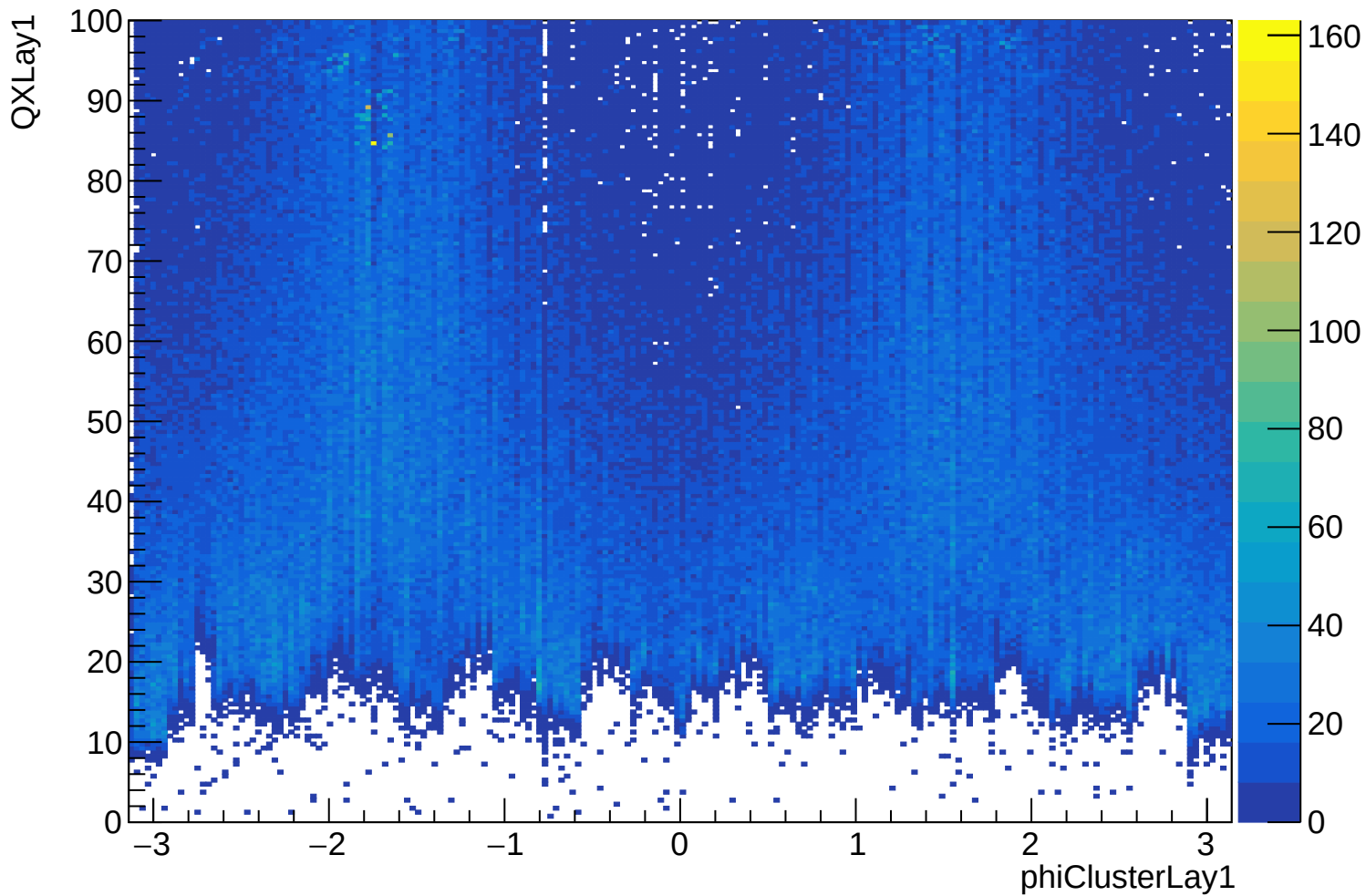
QXLayer1:phiClusterLayer1 {nXStripsLayer1>1}
