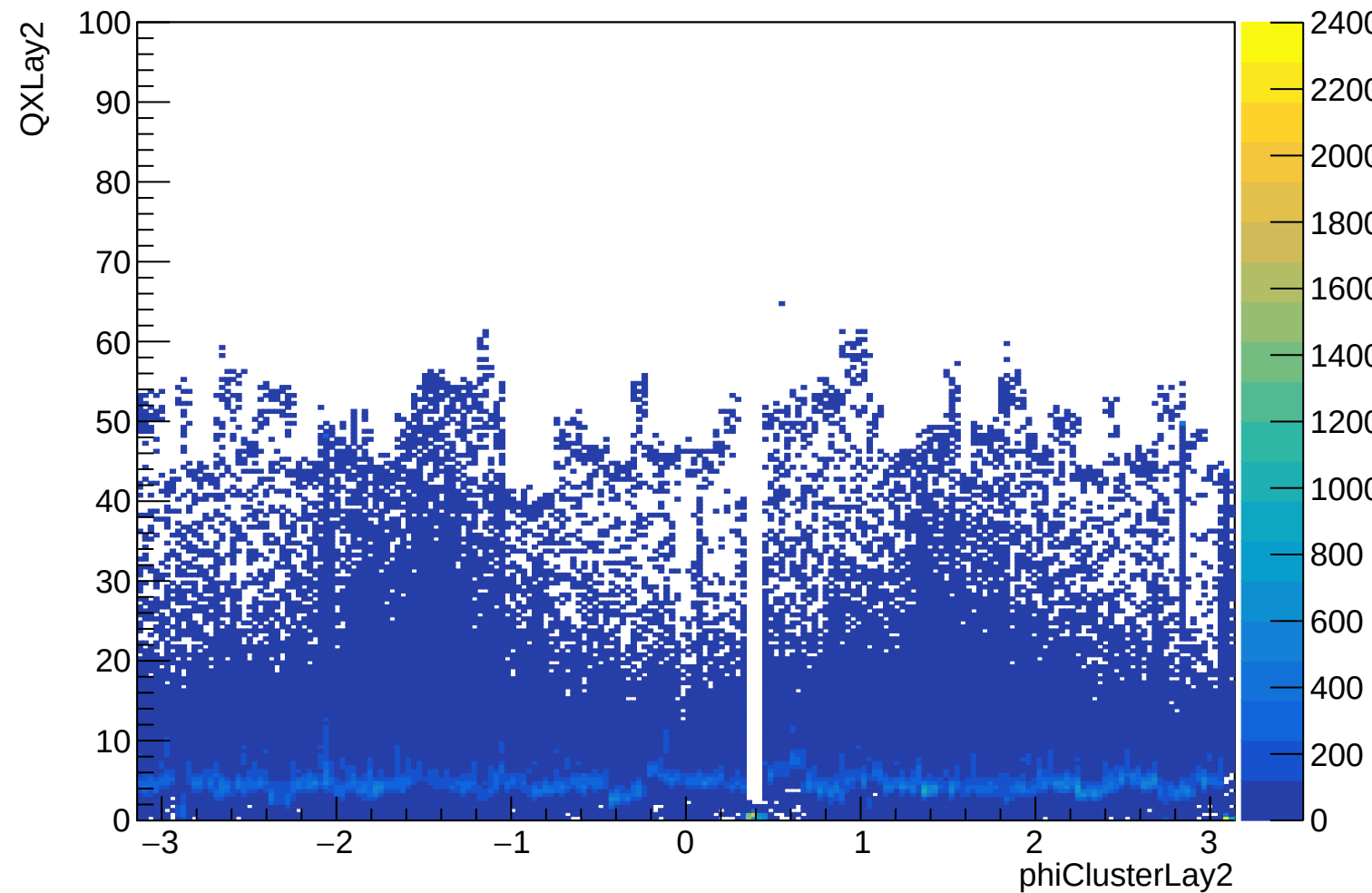
QXLayer2:phiClusterLayer2 {nXStripsLayer2==1}
