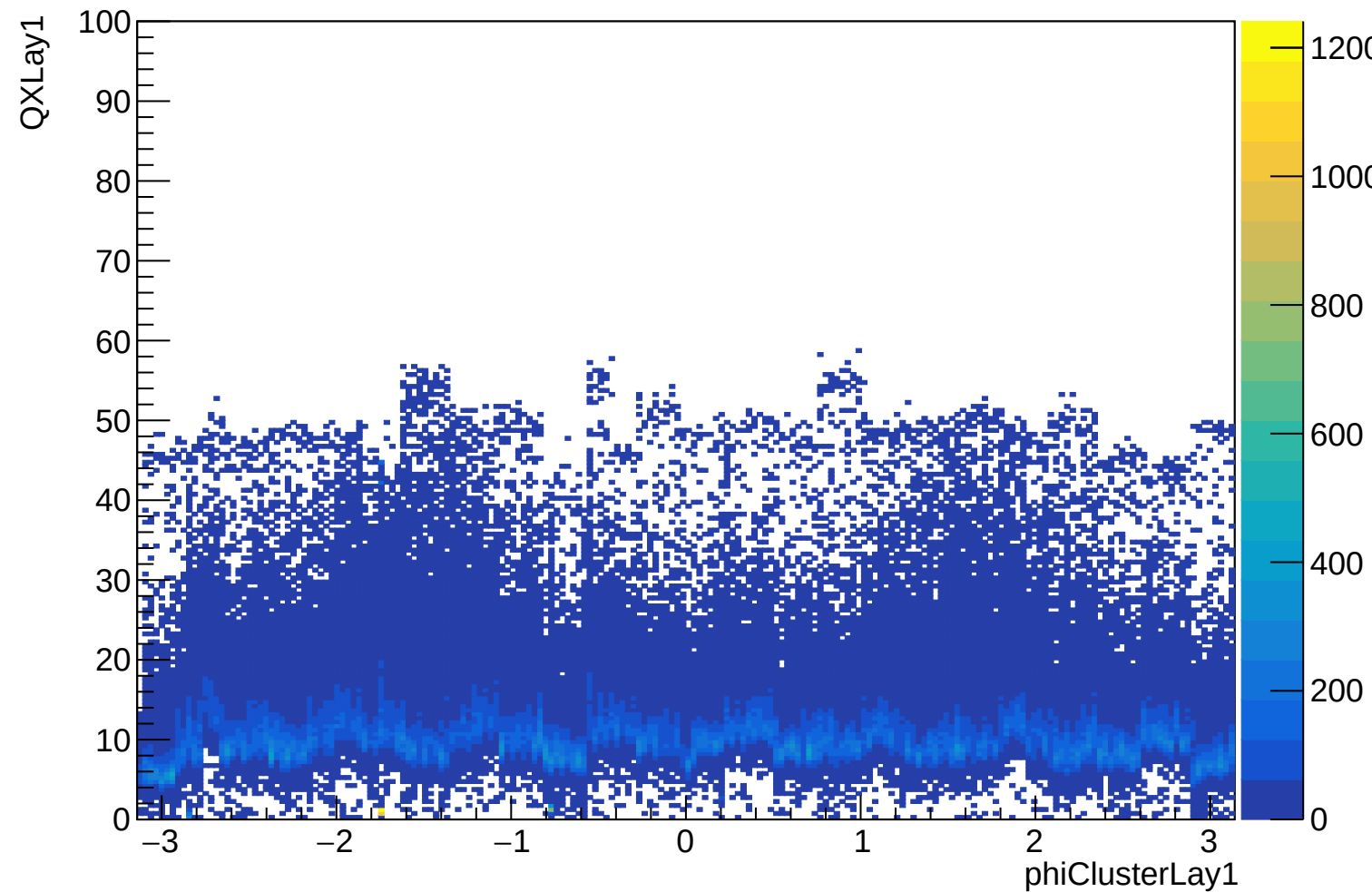
QXLay1:phiClusterLay1 {nXStripsLay1==1}
