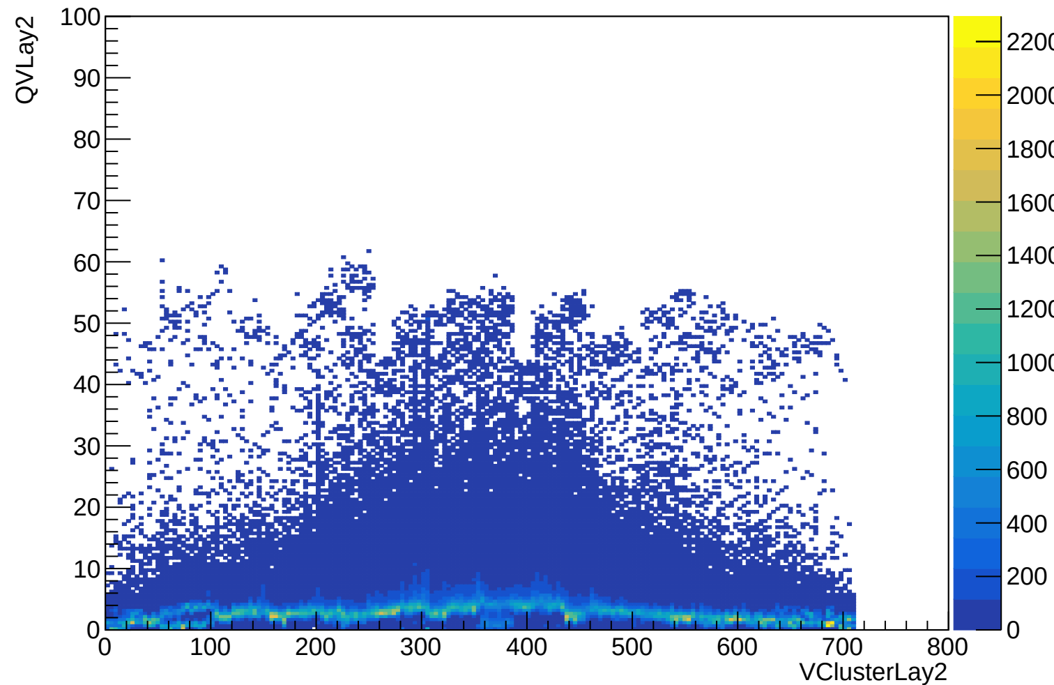
QVLay2:VClusterLay2 {nVStripsLay2==1}
